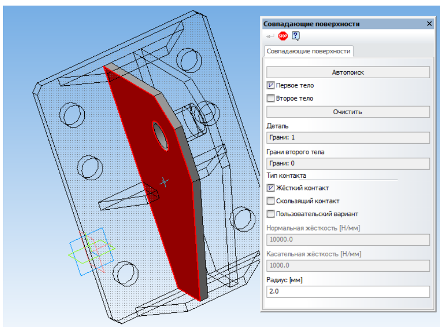
Рис. 2.11. Задание совпадающих поверхностей первого тела
