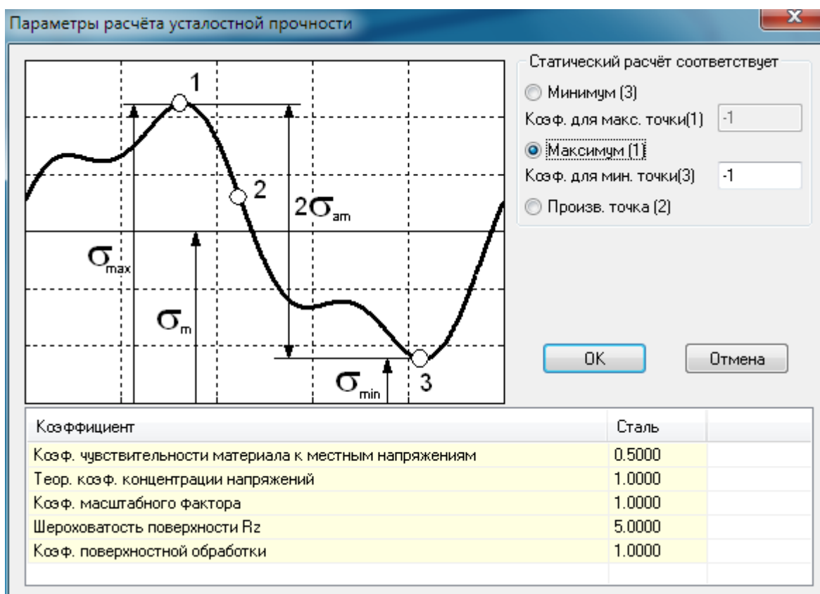
Рис. 2.26. Диалоговое окно Параметры расчёта усталостной прочности
