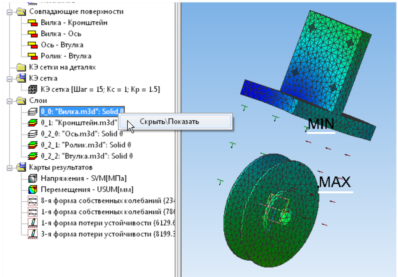
Рис. 2.30. Карта перемещений для сборки с отключёнными слоями
