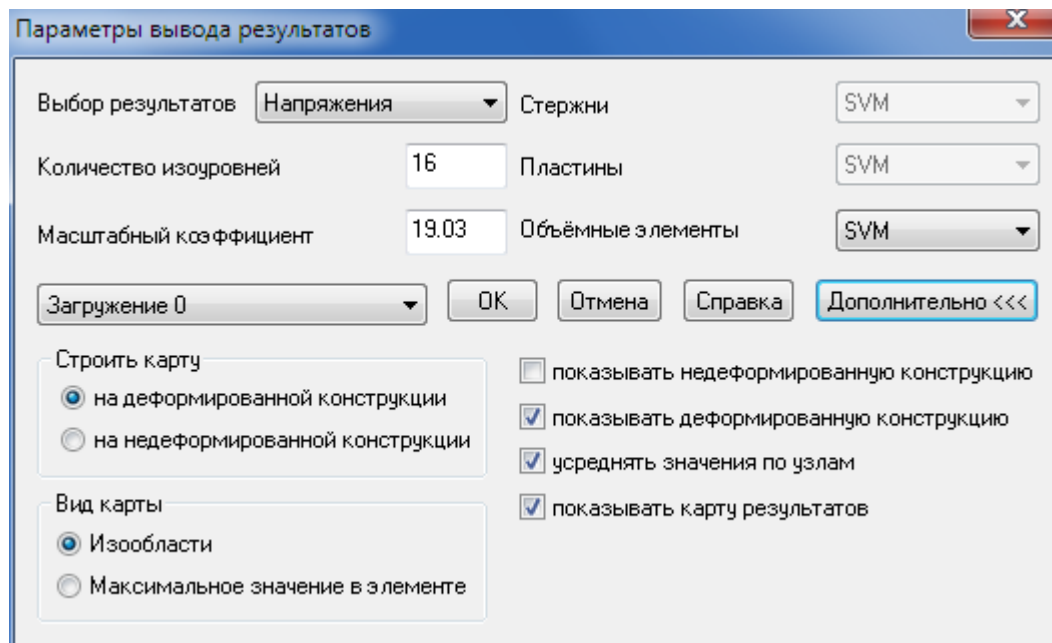
Рис. 2.27. Диалоговое окно Параметры вывода результатов
