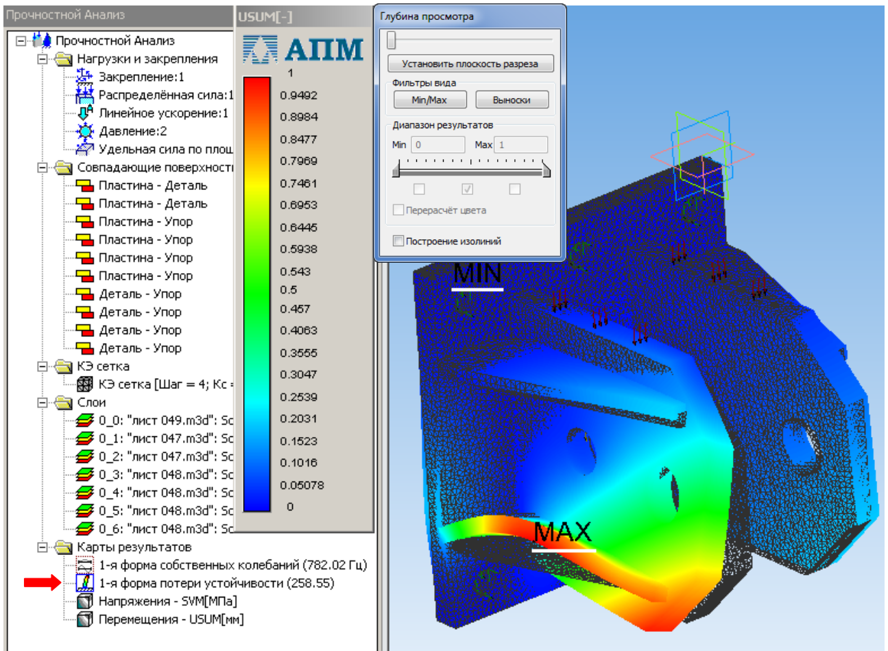
Рис. 2.37. 1-ая форма потери устойчивости
