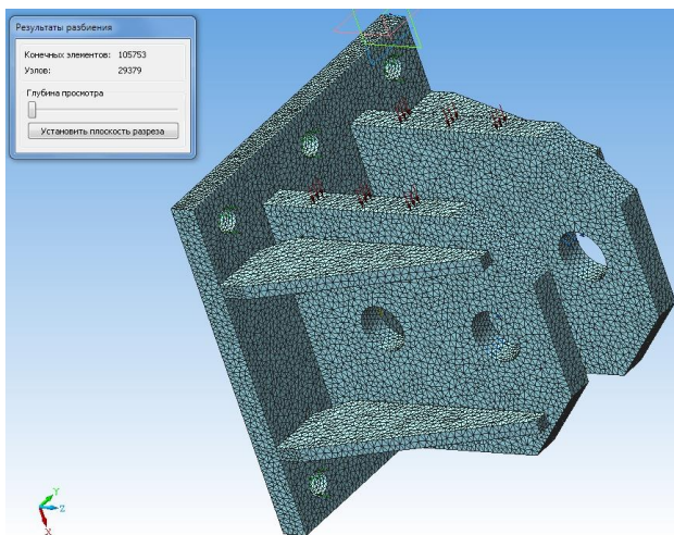
Рис. 2.16. Пример сгенерированной сетки
