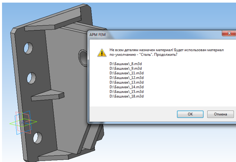
Рис. 1.9. Предупреждение о том, что перечисленным деталям не задан материал из библиотеки
