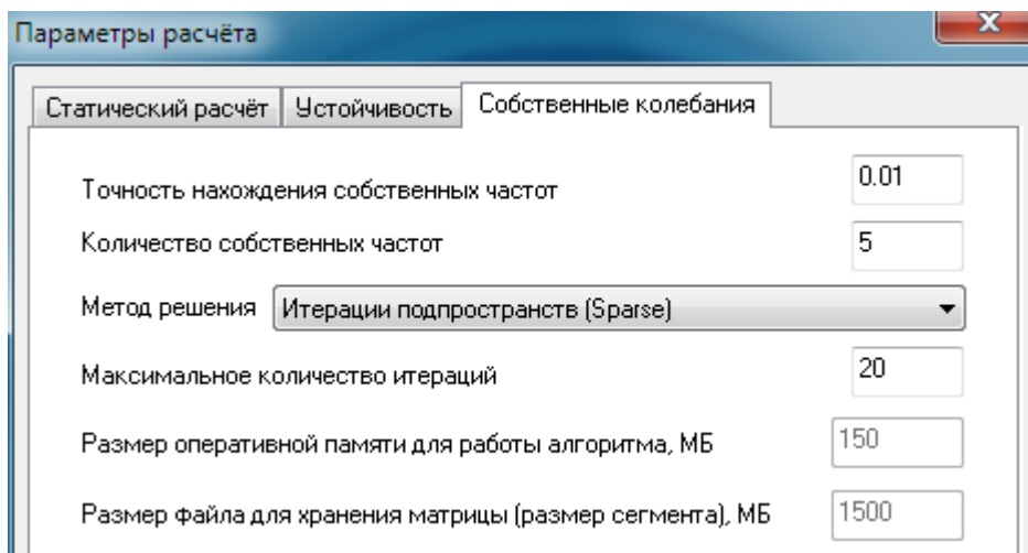
Рис. 2.25. Диалоговое окно Параметры расчета (расчёт собственных колебаний)
