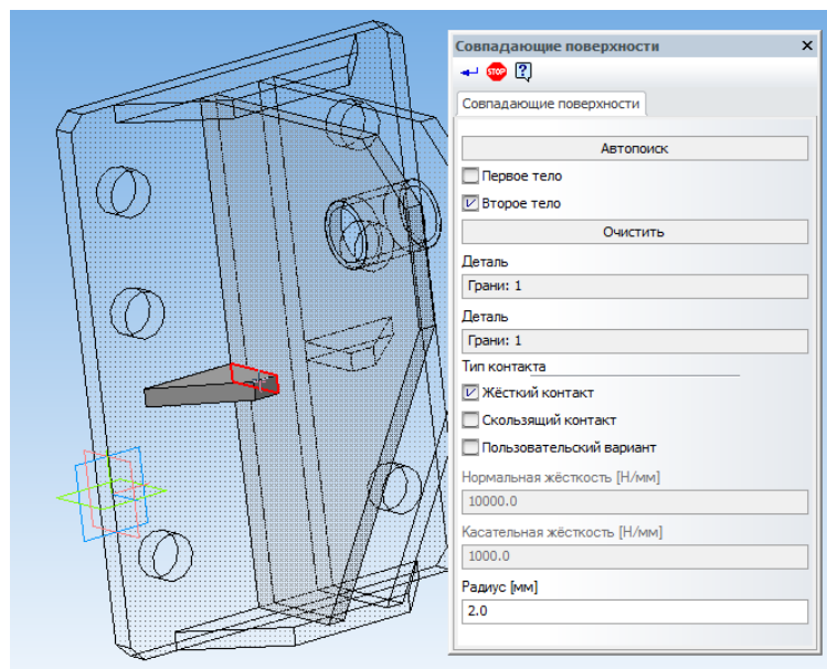
Рис. 2.12. Задание совпадающих поверхностей второго тела
