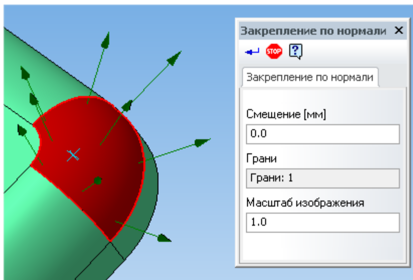
Рис. 2.9. Задание закрепления по нормали
