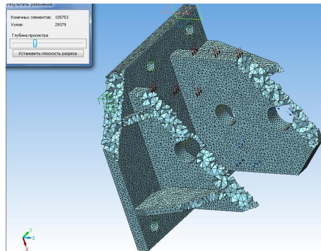
Рис. 2.17. Установка глубины просмотра
