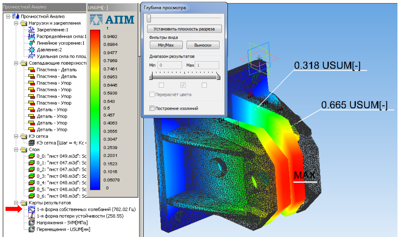
Рис. 2.35. 1-ая форма собственных колебаний
