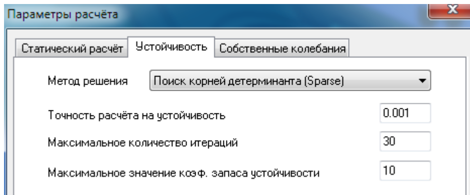
Рис. 2.24. Диалоговое окно Параметры расчета (расчёт устойчивости)
