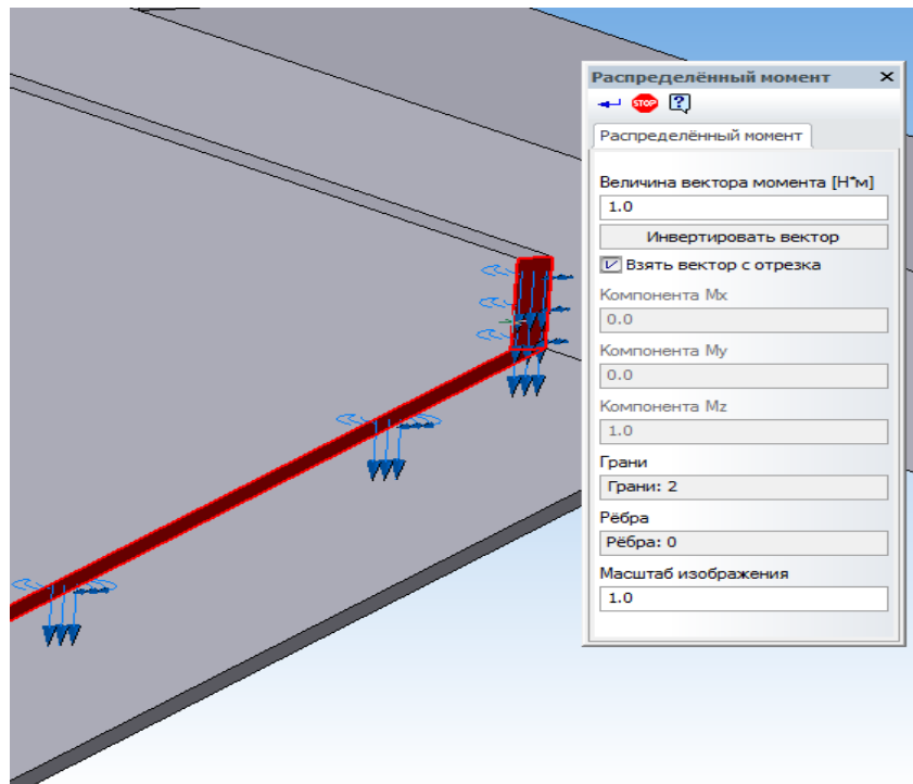
Рис. 2.7. Задание распределенного момента к поверхностям (рёбрам)
