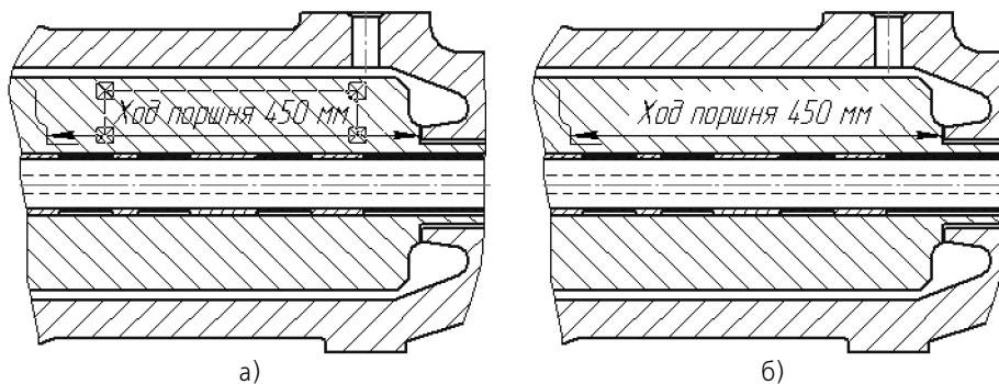
Рис. 142.9. Использование временной ломаной линии в качестве границы области очистки: а) формирование ломаной, б) результат операции
