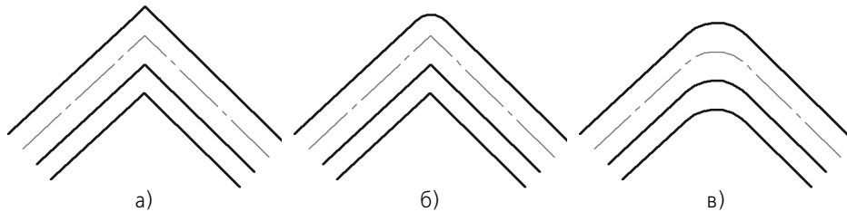
Рис. 123.7. Способы обхода угла в вершине базовой линии: а) обход срезом, б) обход скруглением, в) обход скруглением с одинаковым радиусом
