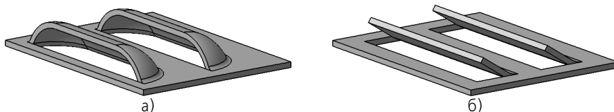
Рис. 42.11. Типы жалюзи
