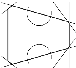
Рис. 125.1. Пример контура, построенного обходом по стрелке
