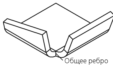
Рис. 38.30. Смежные сгибы
