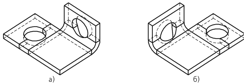
Рис. 40.2. Отверстия, построенные способом По толщине : а) вид детали сразу после создания отверстий, б) результат изменения состояния сгибов
