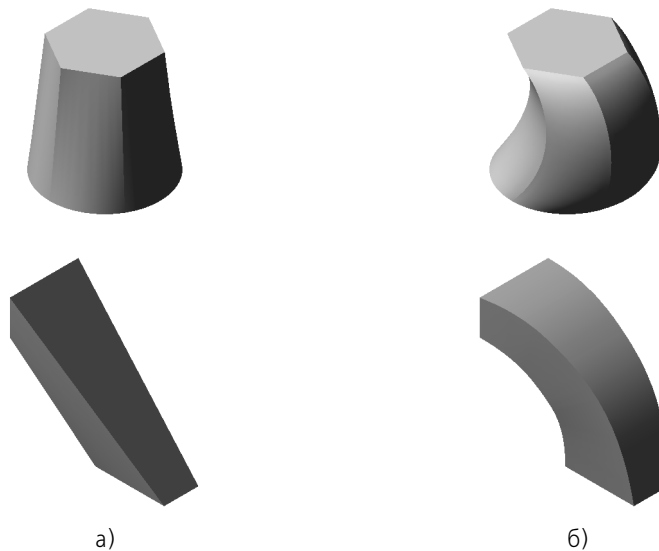
Рис. 26.2. Элементы по сечениям: а) без осевой линии; б) с осевой линией
