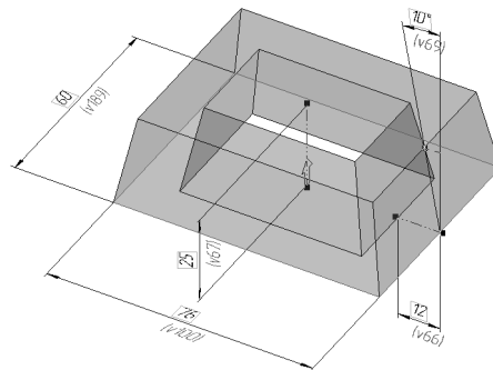
Рис. 19.2. Пример построения элемента выдавливания на основе эскиза
