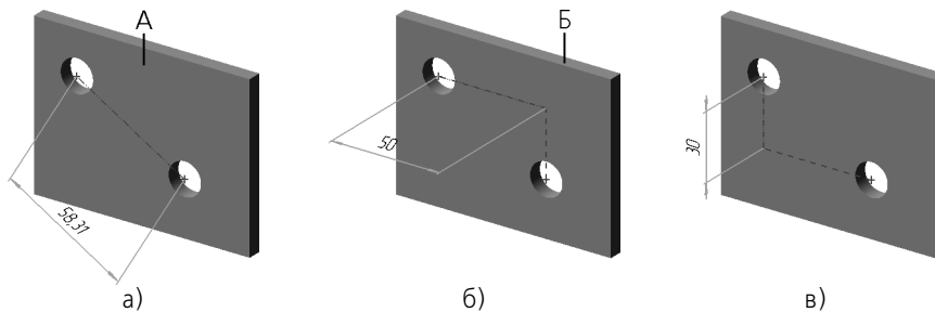
Рис. 64.7. Зависимость положения и значения размера от выбора базовой плоскости: а) базовая плоскость – грань А; б) базовая плоскость – грань Б; в) базовая плоскость – грань В
