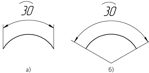
Рис. 128.10. Размер дуги: а) с параллельными выносными линиями, б) с выносными линиями от центра
