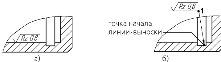
Рис. 133.3. Простановка обозначения шероховатости: а) без полки, б) на полке
