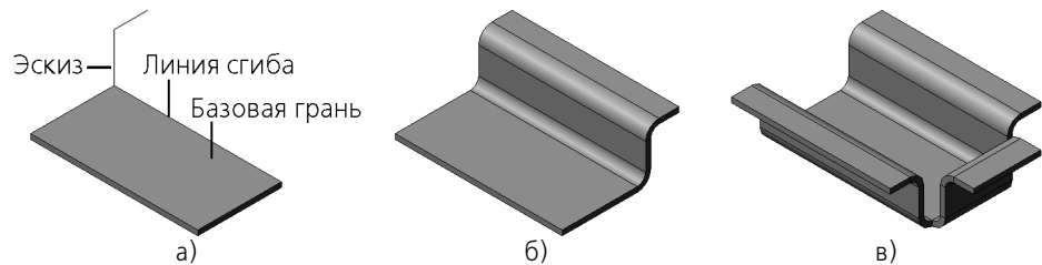
Рис. 38.43. Сгиб по эскизу: а) эскиз сгиба, б) сгиб вдоль одного ребра, в) сгиб вдоль нескольких ребер
