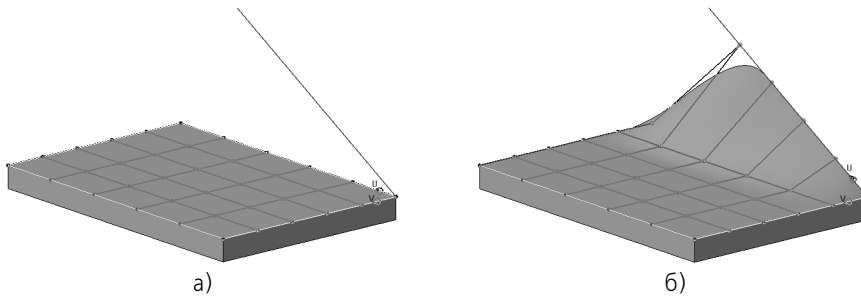
Рис. 49.19. Выравнивание полюсов по направлению: а) исходное состояние грани, б) результат выравнивания
