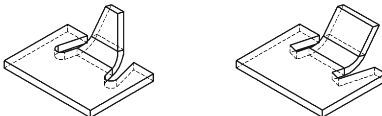
Рис. 38.18. Освобождение сгиба при отличном от нуля угле на сгибе
