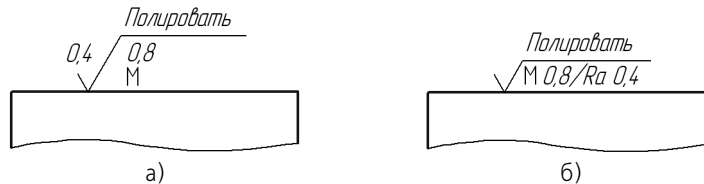
Рис. 133.4. Структура обозначения шероховатости: а) соответствующая предыдущей редакции ГОСТ 2.309–73, б) соответствующая изменению №3, 2003 в ГОСТ 2.309–73
