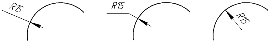
Рис. 129.5. Радиальный размер не от центра
