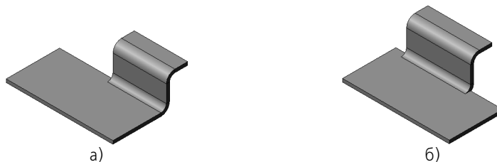
Рис. 38.45. Сгиб На расстояние : а) в одном направлении от плоскости эскиза, б) в двух направлениях
