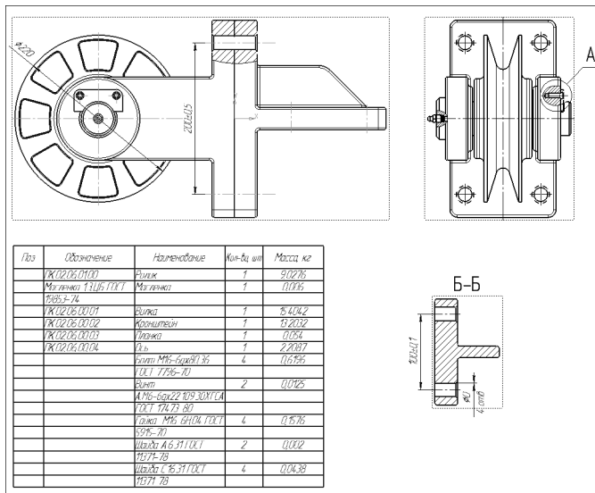
Рис. 178.17. Пример размещения отчета в чертеже
