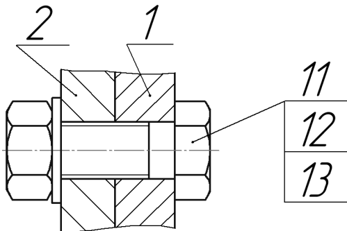
Рис. 133.17. Простановка позиционных линий-выносок
