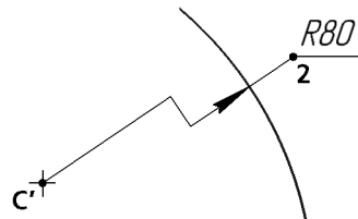
Рис. 129.9. Радиальный размер с надписью, размещенной на полке
