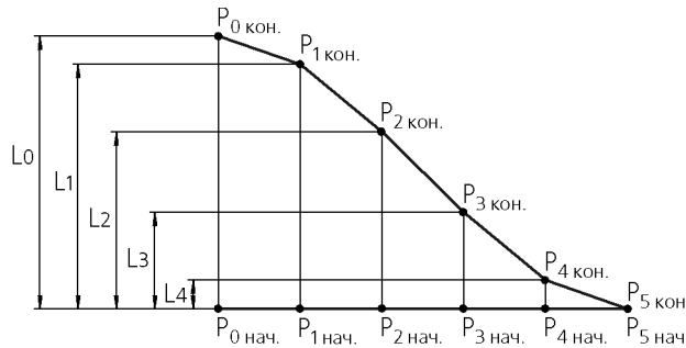
Рис. 49.9. Перемещение полюсов со сглаживанием вида Плавный переход . Первый из выбранных полюсов P_0 перемещается мышью. Последний из выбранных полюсов P_5 наиболее удален от прямой, проходящей в направлении перемещения через полюс P_0 . Перемещение полюса P_5 равно нулю.
