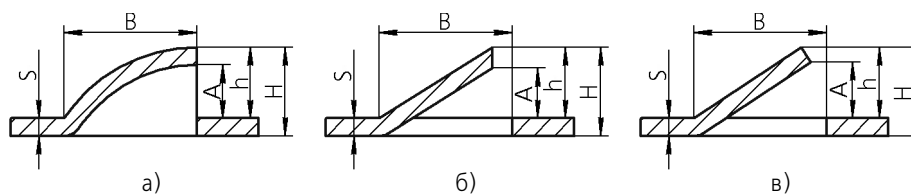
Рис. 42.12. Геометрические параметры жалюзи: а) вытянутых; б) подрезанных с торцем по направлению подрезки; в) подрезанных с торцем по нормали к толщине
