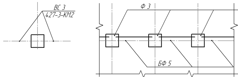
Рис. 134.5. Примеры марки/позиционного обозначения с линией-выноской
