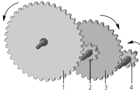
Рис. 79.4. Пример применения сопряжений вращения
