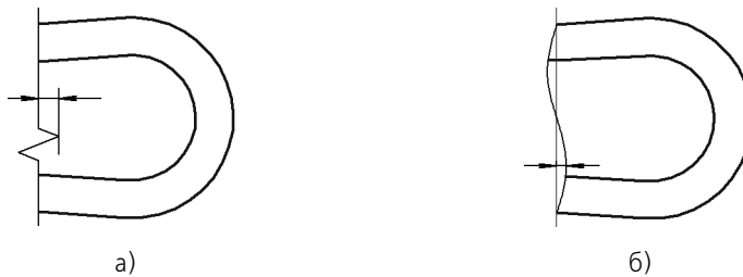
Рис. 150.6. Амплитуда: а) линии с изломом, б) волнистой линии (на рисунке также показана средняя линия)
