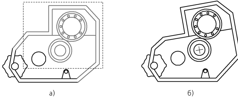
Рис. 140.2. Выполнение деформации поворотом: а) выбор объектов, б) результат операции
