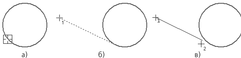
Рис. 122.2. Построение первого отрезка линии касательно к другому объекту: а) указание объекта, б) указание начальной точки отрезка, в) указание конечной точки отрезка
