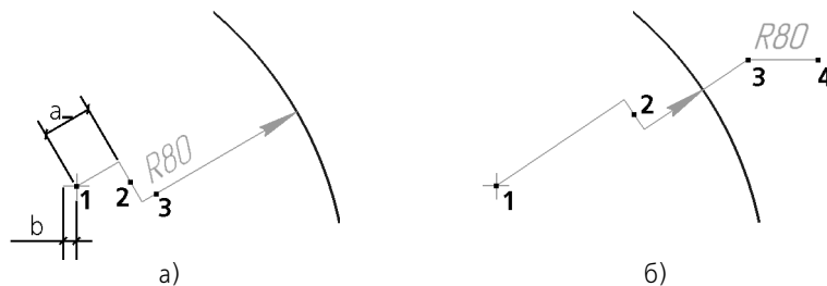
Рис. 129.10. Характерные точки размера с надписью, размещенной: а) вручную, б) на полке
