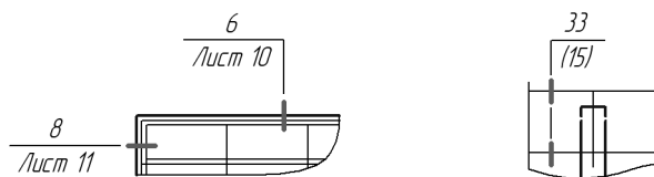
Рис. 134.13. Примеры обозначений узлов в сечении
