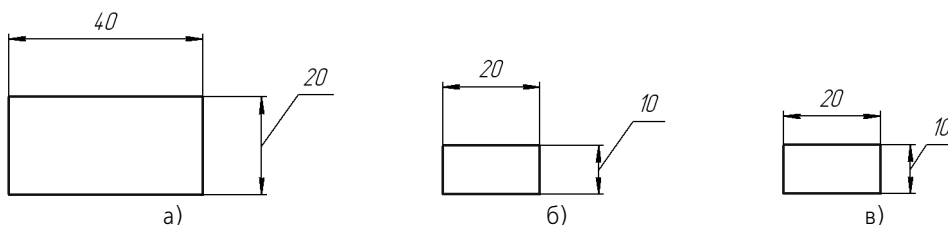
Рис. 139.3. Уменьшение масштаба копий объекта в два раза: а) исходный объект, б) копирование без масштабирования выносных линий, в) копирование с масштабированием выносных линий
