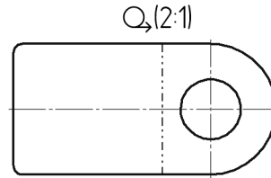
Рис. 41.12. Развертка листового тела
