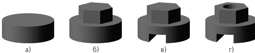
Рис. 22.1. Построение тела: а) новое тело — цилиндр; б) «приклеивание» призмы; в) «вырезание» призмы; г) «вырезание» цилиндра
