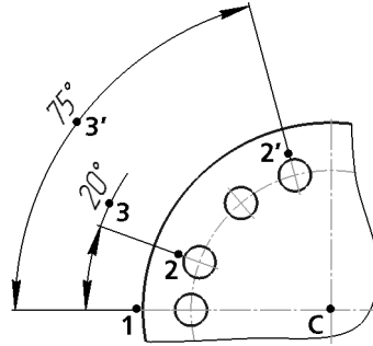
Рис. 130.6. Простановка угловых размеров от общей базы; способ задания сторон угла — по двум отрезкам
