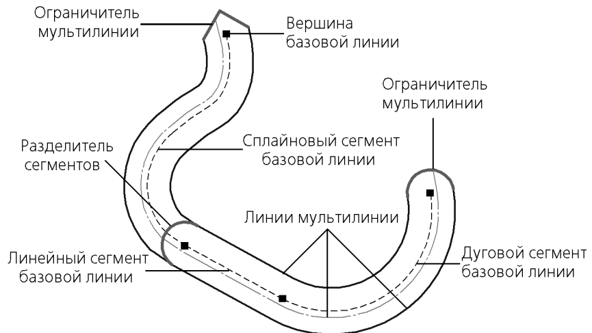
Рис. 123.2. Мультилиния (базовая линия показана пунктиром)
