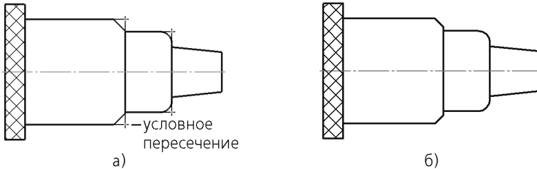
Рис. 126.3. Построение фаски/скругления: а) при включенном построении условного пересечения, б) при выключенном
