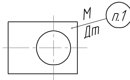
Рис. 133.16. Простановка обозначения маркировки
