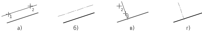
Рис. 133.38. Пример построения автоосевой; способ С указанием границы
