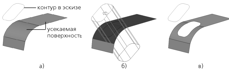
Рис. 48.2. Пример усечения поверхности при помощи контура в эскизе: а) усекаемая поверхность и секущий объект, б) объекты после указания, в) результат усечения
