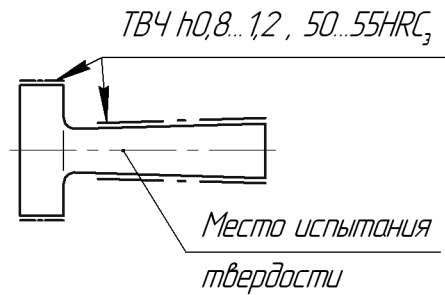
Рис. 133.7. Пример простановки линий-выносок
