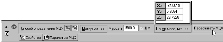
Рис. 75.10. Задание массы и центра масс модели
