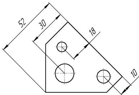
Рис. 128.6. Пример простановки размера между отрезком и точкой
