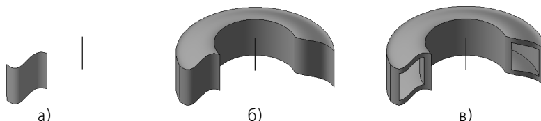
Рис. 24.2. Вращение грани: а) сечение (цилиндрическая грань) и ось, б) сплошной элемент, в) тонкостенный элемент
