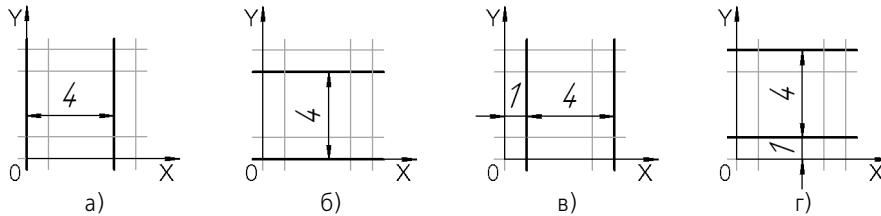
Рис. 256.5. Группы линий, составляющие штриховку Фарфор: а) группа 1, б) группа 2, в) группа 3, г) группа 4
