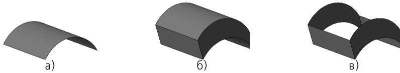
Рис. 47.2. Выдавливание грани: а) сечение (цилиндрическая грань), б) замкнутая поверхность, в) незамкнутая поверхность
