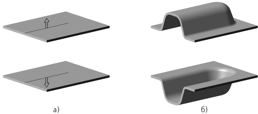
Рис. 42.2. Направление построения штамповочного элемента: а) выбор направления, б) результат построения
