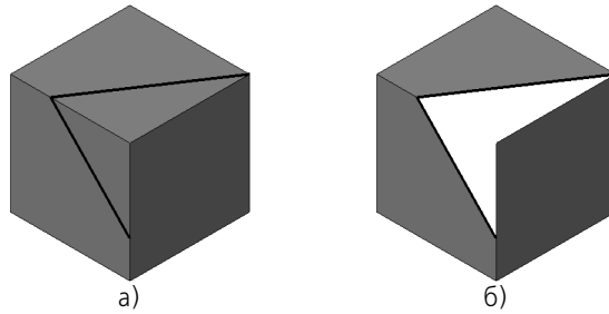
Рис. 48.3. Пример усечения трехгранной поверхности: а) усекаемая поверхность и секущий объект, б) результат усечения
