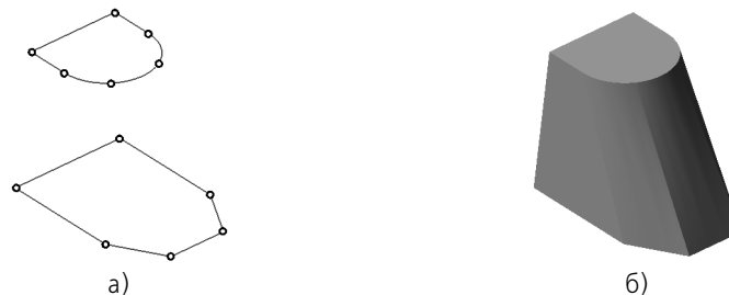
Рис. 26.6. Дуга в верхнем сечении разбита на три части.
