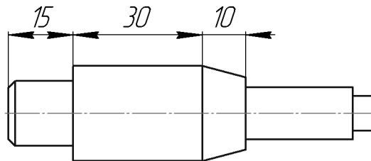
Рис. 128.8. Простановка цепи линейных размеров
