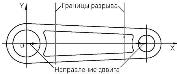
Рис. 150.5. Направление сдвига
