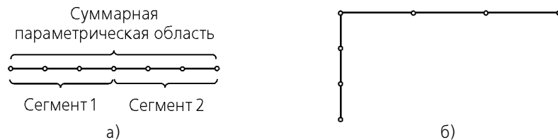
Рис. 45.3. Пример построения группы из 7 точек на ломаной: а) разбиение суммарной параметрической области ломаной на 6 равных участков, б) отображение точек разбиения на сегменты ломаной
