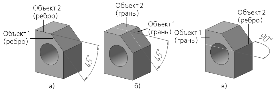
Рис. 64.9. Примеры простановки углового размера: а) между двумя ребрами, б) между двумя гранями, в) между ребром и гранью
