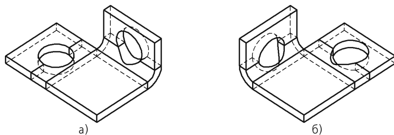
Рис. 40.3. Отверстия, построенные способом На глубину : а) вид детали сразу после создания отверстий, б) результат изменения состояния сгибов
