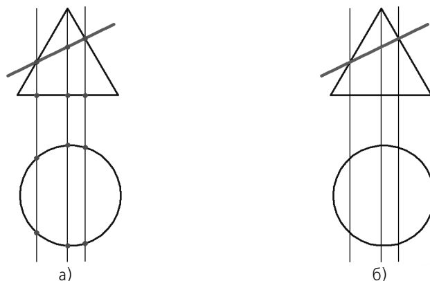
Рис. 114.2. Построение вспомогательных прямых а) с простановкой, б) без простановки вспомогательных точек
