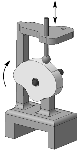
Рис. 79.6. Пример применения сопряжения Кулачок – толкатель
