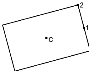
Рис. 119.4. Построение прямоугольника по центру, середине стороны и вершине
