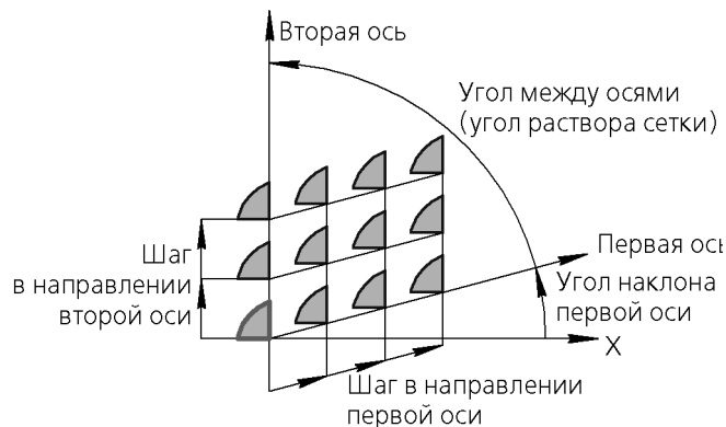
Рис. 51.2. Схема образования параллелограммной сетки
