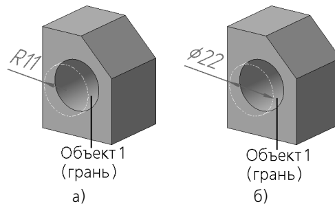
Рис. 64.11. Примеры простановки размеров к грани детали: а) радиального, б) диаметального
