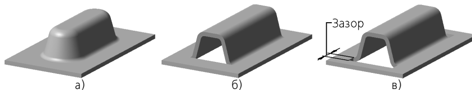
Рис. 42.10. Типы обработки концов буртика
