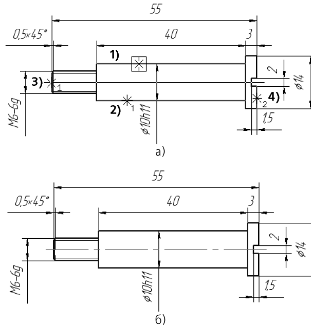
Рис. 133.42. Построение автоосевой на чертеже способом С указанием границы : а) указание объектов для построения автоосевой, б) построенная автоосевая
