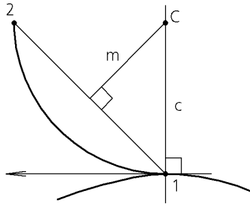
Рис. 46.6. Определение центральной точки дуги и радиуса
