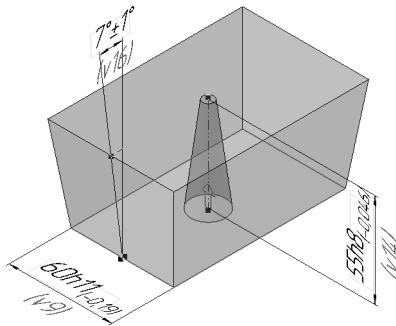
Рис. 68.1. Отображение индивидуальных допусков при создании элемента выдавливания
