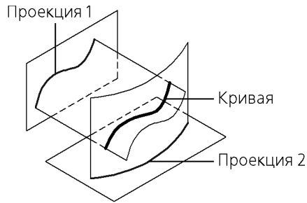
Рис. 46.23. Построение кривой по двум проекциям
