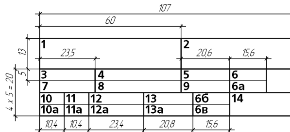
Рис. 259.2. Структура и размеры дополнительного штампа
