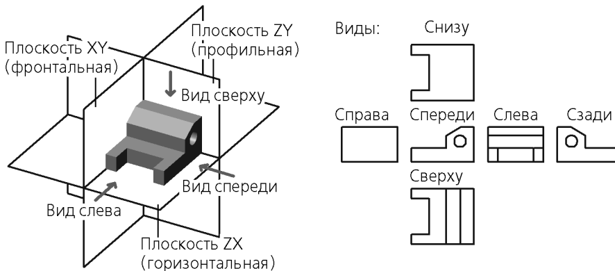
Рис. 20.1. Положение детали относительно координатных плоскостей
