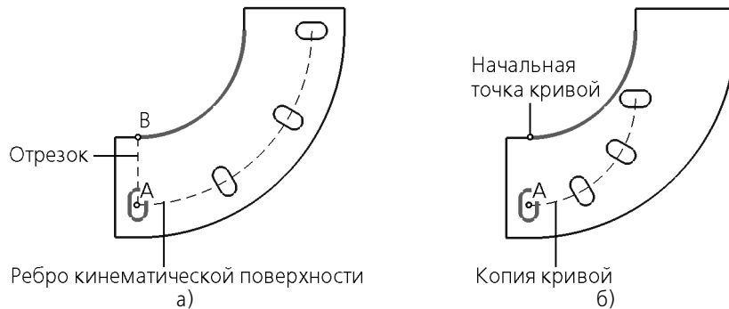
Рис. 53.2. Схема копирования операции выдавливания вдоль всей направляющей с сохранением ориентации (траектория и копируемый объект выделены):
