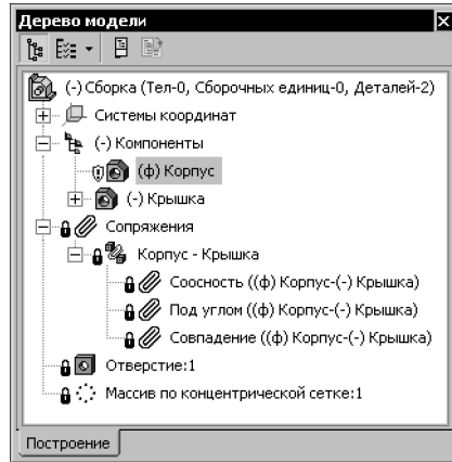
Рис. 84.2. Объекты модели, заблокированные в результате наложения запрета редактирования на один из компонентов
