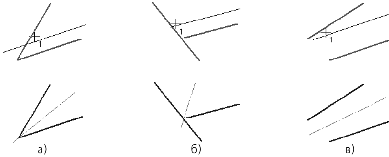
Рис. 133.36. Примеры построения автоосевой
