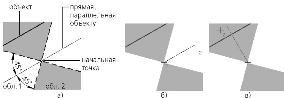
Рис. 122.1. Построение отрезка параллельно/перпендикулярно прямолинейному объекту
