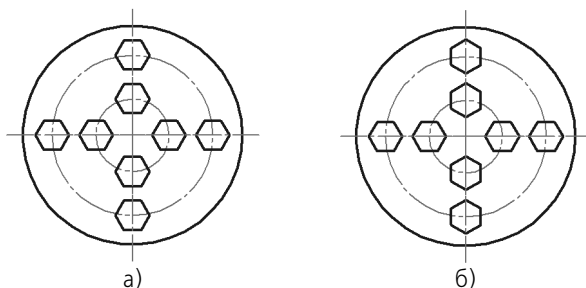
Рис. 138.10. Копирование по концентрической сетке: а) без доворота до радиального направления, б) с доворотом до радиального направления
