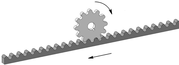
Рис. 79.5. Пример применения сопряжения Вращение – перемещение
