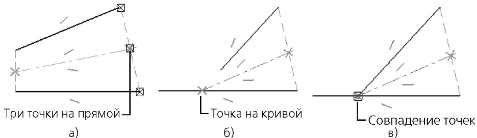
Рис. 212.1. Ограничения, наложенные на автоосевую при различном расположении отрезков
