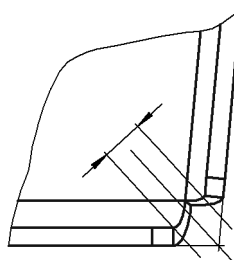
Рис. 38.36. Максимальный зазор при замыкании встык
