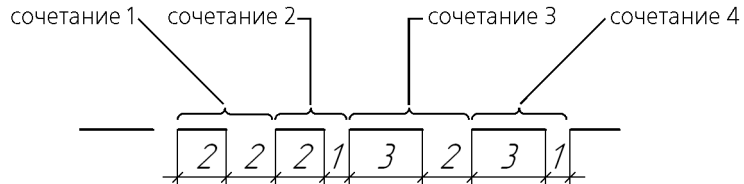
Рис. 256.9. Сочетания штрихов и промежутков в прерывистых линиях штриховки Термопласт
