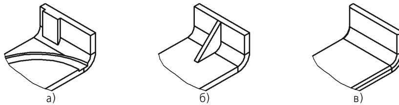
Рис. 41.7. Примеры формообразующих и конструктивных элементов, делающих невозможным разгибание сгиба: а) приклеенный и вырезанный элементы, б) ребро жесткости, в) фаска
