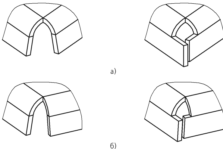
Рис. 38.37. Замыкание с перекрытием (исходное состояние детали и результат операции): а) замыкаемый угол острый, б) замыкаемый угол тупой
