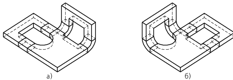
Рис. 40.7. Вырезы, построенные способом На глубину : а) вид детали сразу после создания вырезов, б) результат изменения состояния сгибов
