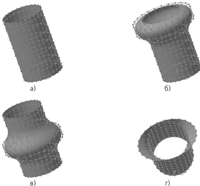
Рис. 49.14. Масштабирование полюсов: а) исходное состояние грани, б) равномерное масштабирование, в) масштабирование в плоскости, г) масштабирование по оси
