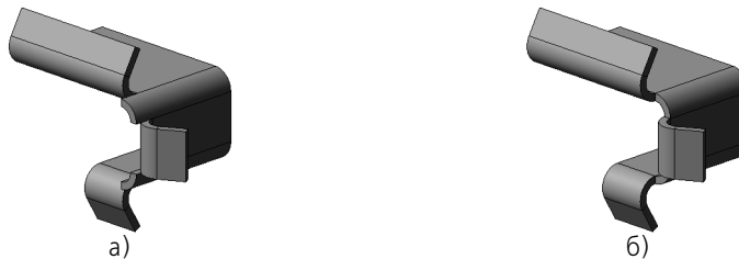
Рис. 38.53. Сгиб вдоль цепочки ребер, соединенных сгибами: а) без освобождения угла, б) с освобождением угла
