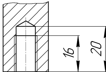
Рис. 128.7. Простановка линейных размеров от общей базы
