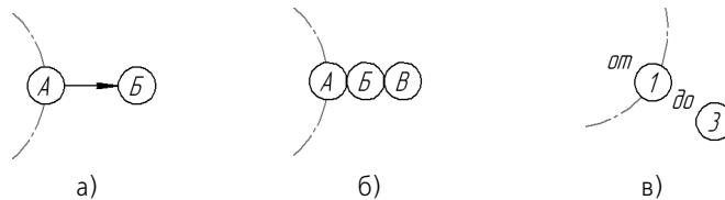
Рис. 134.31. Элементы дополнительных обозначений круговой оси: а) указатель ориентации, б) марка, в) текст
