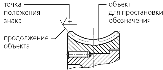
Рис. 133.2. Простановка обозначения шероховатости на продолжении объекта
