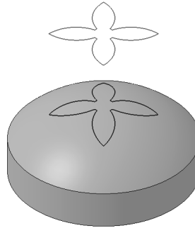
Рис. 46.39. Проекция эскиза на грань тела
