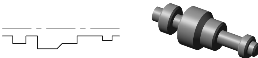
Рис. 24.5. Построение элемента вращения с плоскими торцами
