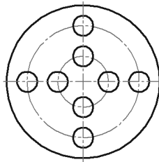
Рис. 138.9. Пример копирования по концентрической сетке
