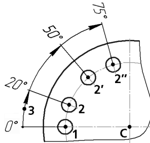
Рис. 130.8. Простановка угловых размеров с общей размерной линией; способ задания сторон угла — по трем точкам
