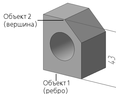
Рис. 64.8. Пример простановки линейного размера от отрезка до точки
