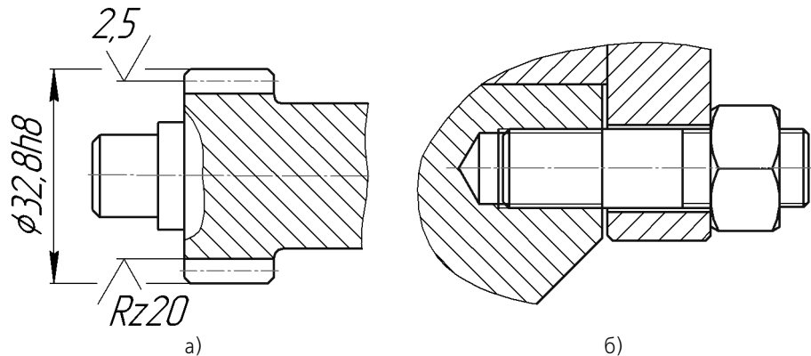
Рис. 142.10. Удаление части изображения: а) выносной линии размера, б) крепежного элемента (шпильки)
