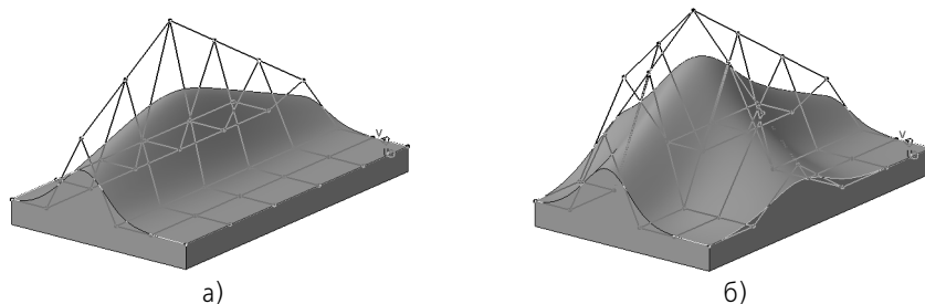
Рис. 49.4. Пропорциональное перемещение полюсов: а) в ряду по направлению U , б) в рядах по направлениям U и V
