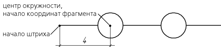
Рис. 255.9. Положение окружности относительно начала штриха
