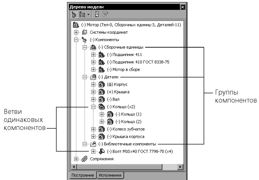
Рис. 17.3. Структура сборки с отображением групп
