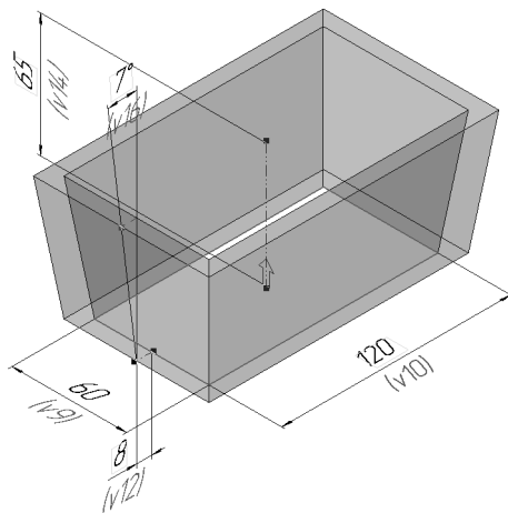
Рис. 64.1. Пример построения элемента выдавливания
