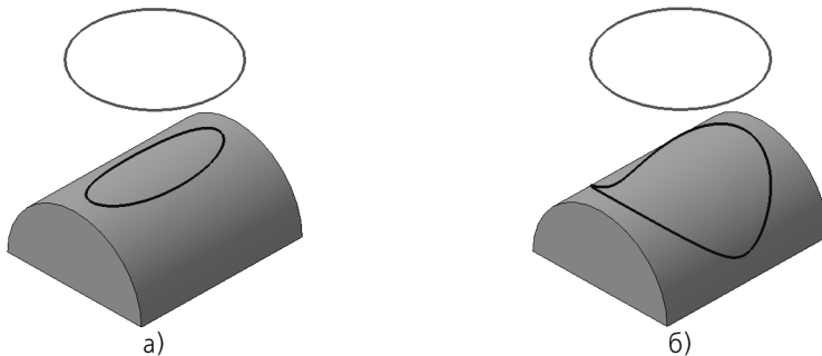
Рис. 46.41. Пример построения проекции линии эскиза на цилиндрическую поверхность: а) проецирование линии эскиза по нормали к поверхности; б) проецирование линии эскиза перпендикулярно плоскости эскиза
