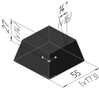
Рис. 50.8. Пример отображения размеров, соответствующих переменным операции выдавливания
