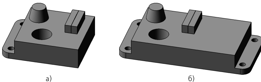
Рис. 56.1. Зеркальное копирование объектов: а) исходная деталь (плоскость симметрии для копирования показана условно), б) результат копирования основания и лапки относительно средней плоскости прямоугольного выступа
