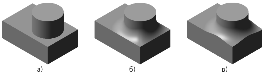
Рис. 30.4. Скругление: а) исходные элементы, б) скругление с сохранением кромки, в) скругление без сохранения кромки
