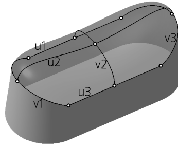
Рис. 47.17. Поверхность по сети кривых. u_1, u_2, u_3 – кривые направления U ; v_1, v_2, v_3 – кривые направления V . Узлы сети отмечены кружками
