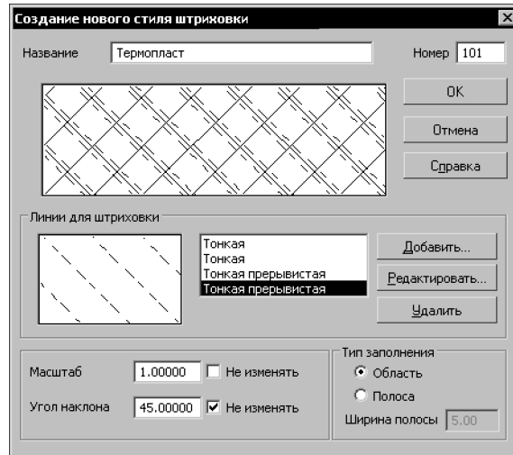
Рис. 256.12. Создание третьей и четвертой групп линий
