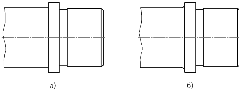
Рис. 126.5. Построение скругления: а) исходное изображение, б) результат построения
