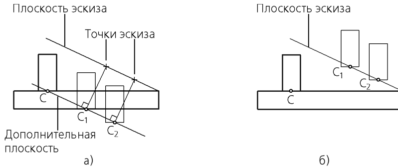
Рис. 54.2. Задание позиций экземпляров массива: а) при включенной опции Проецировать ; б) при отключенной опции Проецировать
