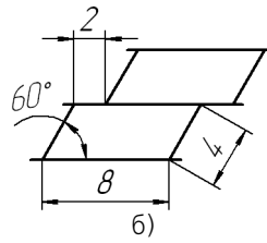
Рис. 256.16. Стил штриховки Гранит: а) образец штриховки, б) размер и расположение элементов штриховки
