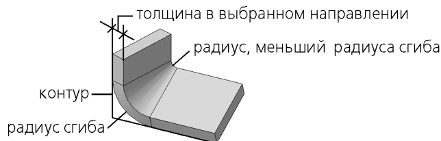
Рис. 37.2. Радиусы сгиба обечайки с уклоном
