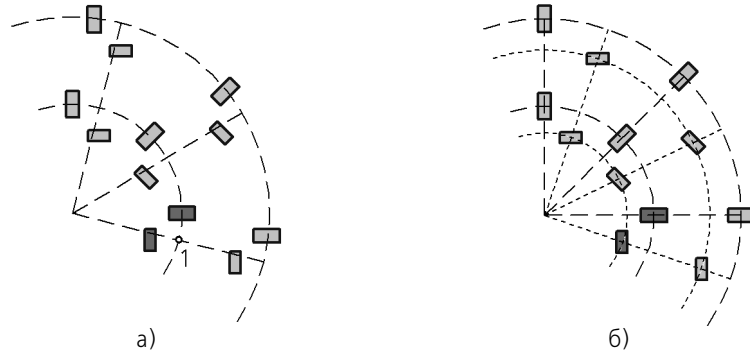
Рис. 52.3. Массив группы объектов по концентрической сетке с доворотом: а) в качестве базовой указана точка 1, б) базовая точка не указана
