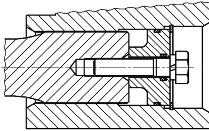
Рис. 133.44. Пример использования волнистой линии
