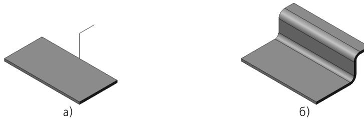
Рис. 38.44. Сгиб По ребру : а) исходное состояние модели и эскиз сгиба, б) результат построения
