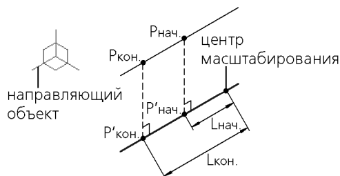
Рис. 49.16. Перемещение полюса при масштабировании по направлению, направляющим объектом является ось X
