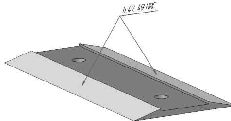
Рис. 65.4. Пример простановки линии-выноски
