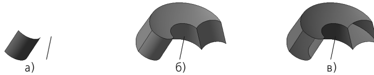
Рис. 47.5. Вращение грани: а) сечение (цилиндрическая грань) и ось, б) замкнутая поверхность, в) незамкнутая поверхность
