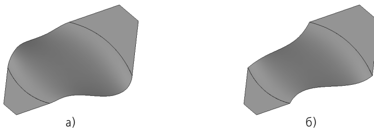
Рис. 47.26. Боковые ребра поверхности соединения: а) продолжения боковых ребер соединяемых поверхностей; б) перпендикулярны границам
