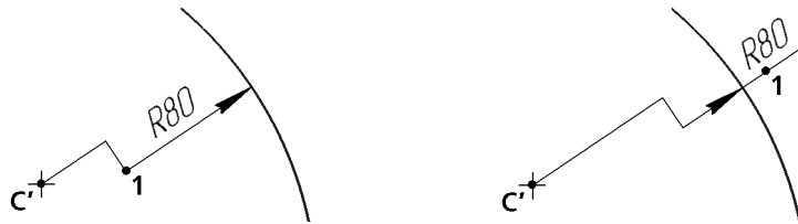
Рис. 129.8. Радиальные размеры с изломом с автоматически размещенной надписью
