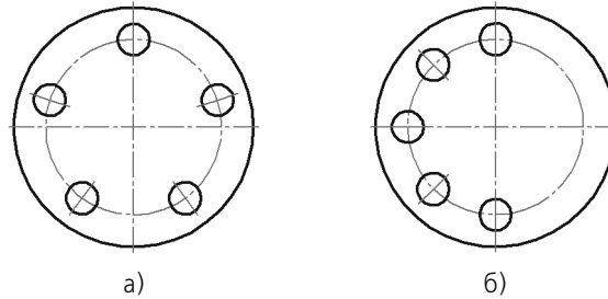
Рис. 138.11. Режим копирования: а) вдоль всей окружности, б) с угловым шагом 45^\circ
