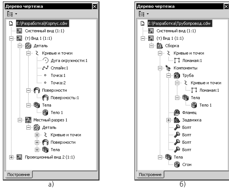
Рис. 154.3. Деревя чертежа с ассоциативными видами: а) детали, б) сборки
