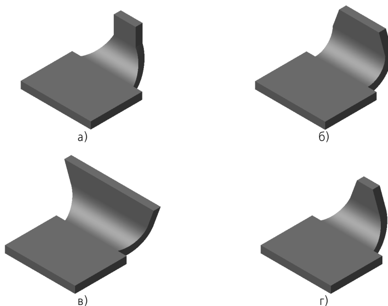
Рис. 38.15. Управление боковыми сторонами сгиба: а) углы на сгибе, б) уклон боковых сторон продолжения сгиба, в), г) углы на сгибе и уклон боковых сторон продолжения
