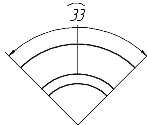
Рис. 128.11. Пример простановки размера дуги с указателем от текста к дуге
