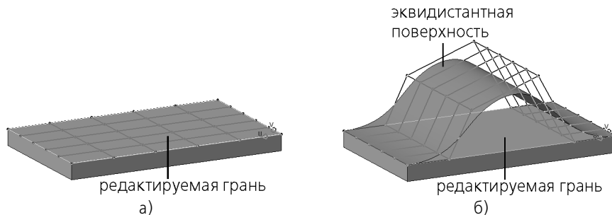
Рис. 49.26. Построение слайновой формы на эквидистантной поверхности: а) редактируемая грань, б) эквидистантная поверхность и редактируемая грань
