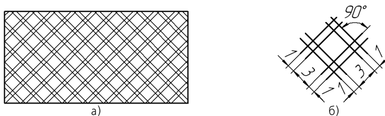
Рис. 256.14. Стиль штриховки Изоляционный слой: а) образец штриховки, б) размер и расположение элементов штриховки
