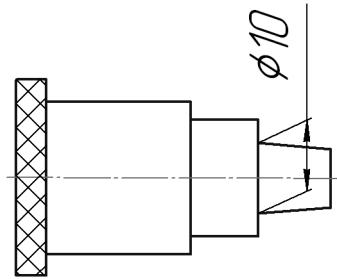
Рис. 128.4. Пример простановки размера с наклонными выносными линиями
