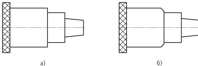
Рис. 126.1. Построение фаски: а) исходное изображение, б) результат выполнения команды
