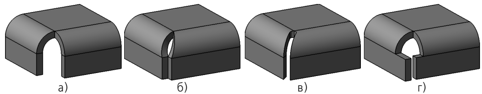
Рис. 38.29. Замыкание угла: а) исходное состояние детали, б), в), г) варианты замыкания угла
