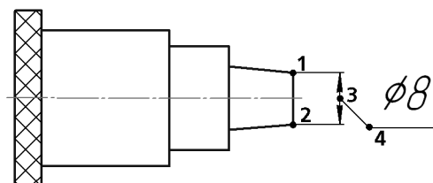
Рис. 128.2. Линейный размер на полке
