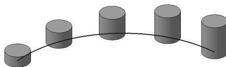
Рис. 50.7. Пример изменения размеров экземпляров массива операции выдавливания: для каждого экземпляра задано новое значение расстояния выдавливания
