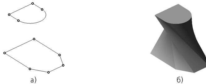
Рис. 26.5. Автоматическое соединение сечений с разной топологией
