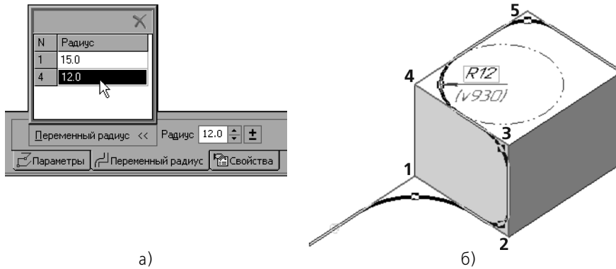
Рис. 46.42. Пример построения контура с переменным радиусом скруглений: а) задание значения радиуса в таблице; б) отображение скруглений на фантоме контура
