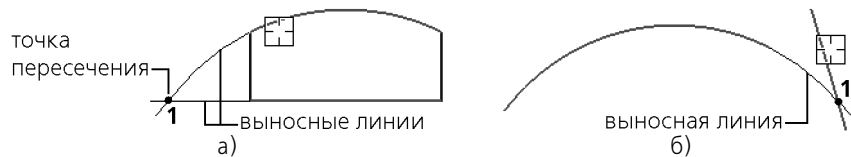
Рис. 133.54. Условное пересечение: а) для продолжений двух объектов; б) для объекта и продолжения другого объекта
