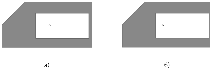
Рис. 60.6. Варианты расположения центра масс плоской грани: а) при включенной опции Только внешний контур , б) при отключенной опции Только внешний контур
