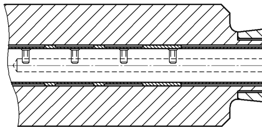
Рис. 138.3. Пример копирования по кривой
