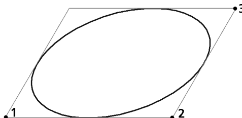
Рис. 117.5. Эллипс по трем вершинам габаритного параллелограмма
