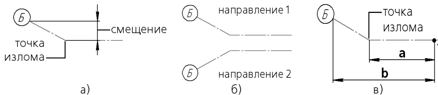
Рис. 134.26. Параметры выступа координационной оси: а) смещение, б) направление, в) смещение излома
