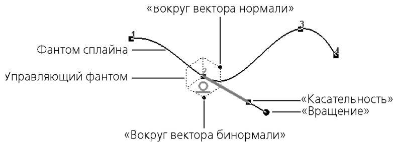
Рис. 46.13. Управляющий фантом при управлении ориентацией касательной и касательностью
