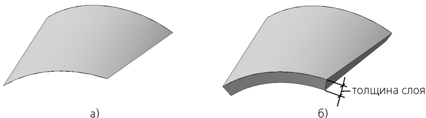
Рис. 28.1. Придание толщины грани поверхности: а) исходная грань, б) добавление слоя материала в одном направлении
