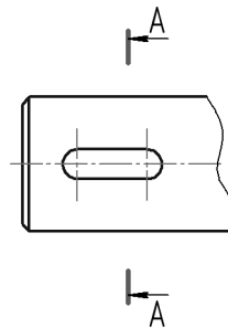
Рис. 133.25. Простановка линии разреза
