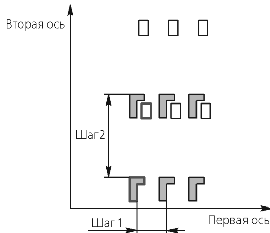
Рис. 57.2. Размещение экземпляров массива по образцу согласно параметрам массива-образца
