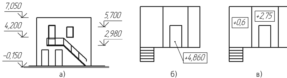
Рис. 132.1. Размер высоты: а) для вида спереди или разреза, б) для вида сверху с линией-выноской, в) для вида сверху непосредственно на изображении
