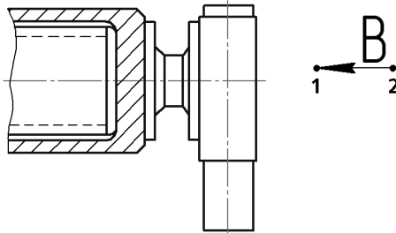
Рис. 133.22. Простановка стрелки направления взгляда
