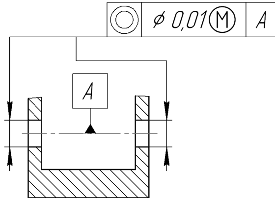
Рис. 133.31. Простановка допуска расположения поверхностей
