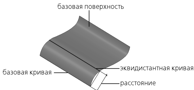
Рис. 46.34. Эквидистантная кривая, построенная способом Смещение вдоль поверхности
