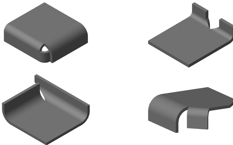
Рис. 38.42. Примеры смежных сгибов, замыкание угла между которыми невозможно
