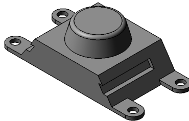
Рис. 22.2. Бобышка и лапки приклеены к телу, пазы и отверстия — вырезаны из него
