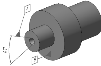
Рис. 65.3. Пример простановки обозначения базы
