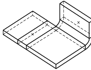
Рис. 40.1. Исходное состояние детали. Центры будущих отверстий (расположенные на невидимых гранях) обозначены «крестиками»
