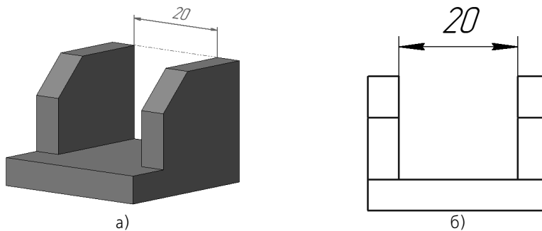
Рис. 156.1. Линейный размер в модели (а) и соответствующий ему проекционный размер в ассоциативном виде (б)
