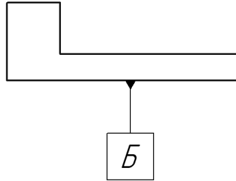
Рис. 133.28. Пример простановки обозначения базы
