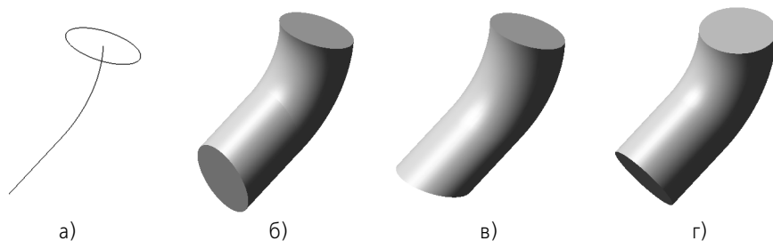
Рис. 25.2. Кинематический элемент: а) эскизы сечения и траектории, б) перемещение сечения с сохранением угла наклона, в) перемещение сечения параллельно самому себе, г) перемещение сечения ортогонально траектории.
