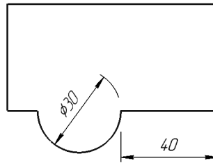
Рис. 127.10. Пример простановки линейного и диаметрального размеров с зазором
