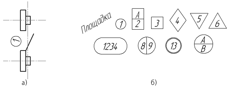
Рис. 134.3. Марка/позиционное обозначение без линии-выноски а) пример использования, б) типы формы обозначения
