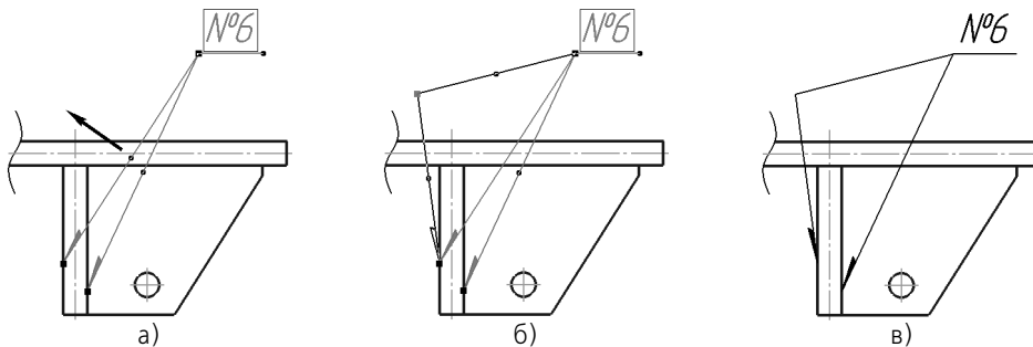
Рис. 133.12. Формирование излома выноски
