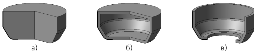
Рис. 24.3. Построение сфероида и тороида (сечение – эскиз – выделено утолщенной линией) а) сфероид сплошной, б) сфероид тонкостенный, в) тороид
