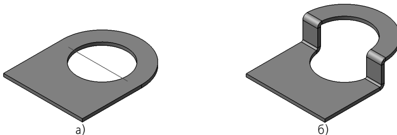
Рис. 38.27. Подсечка в детали с отверстием: а) положение линии сгиба, б) результат построения
