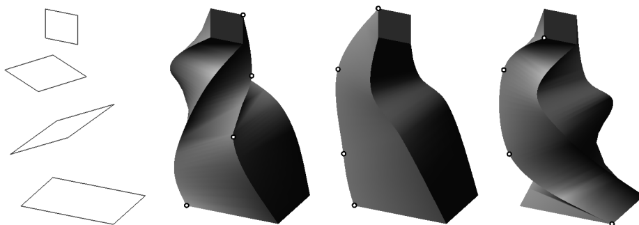
Рис. 26.4. Элементы, образованные путем соединения разных точек одинаковых сечений (соединенные точки выделены)
