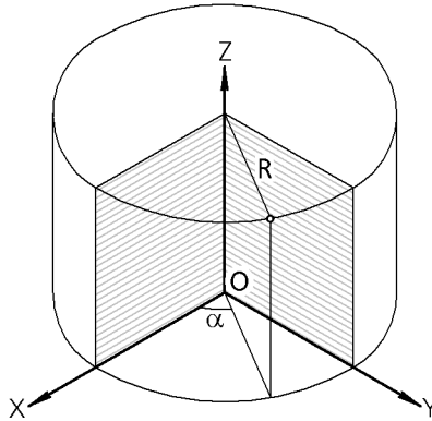
Рис. 45.8. Построение точки по цилиндрическим координатам; XYZ – система координат точки
