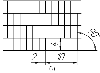
Рис. 256.15. Стил штриховки Соли: а) образец штриховки, б) размер и расположение элементов штриховки
