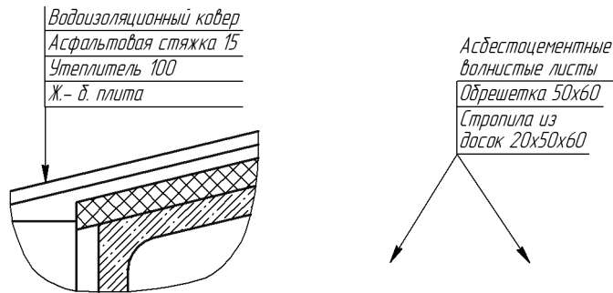
Рис. 134.20. Примеры выносной надписи
