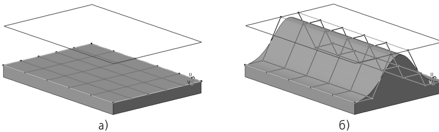
Рис. 49.20. Выравнивание полюсов по плоскому объекту: а) исходное состояние грани, б) результат выравнивания
