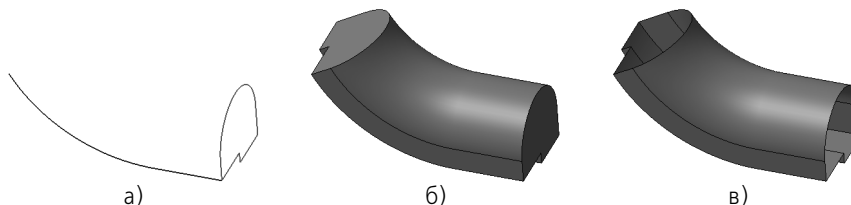
Рис. 47.8. Кинематическая поверхность: а) сечение и траектория, б) замкнутая поверхность, в) незамкнутая поверхность
