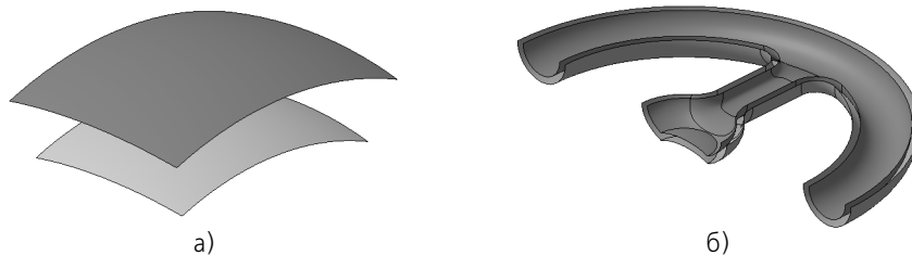
Рис. 47.27. Эквидистантная поверхность: а) базовая поверхность — грань поверхности; б) базовая поверхность — совокупность граней
