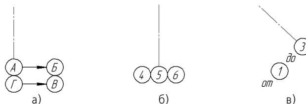
Рис. 134.23. Элементы дополнительных обозначений: а) указатель ориентации, б) марка, в) текст
