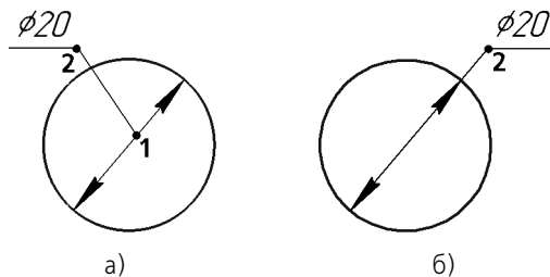
Рис. 129.2. Диаметральные размеры с надписью, размещенной на полке: а) линия-выноска не совпадает с размерной линией, б) линия-выноска совпадает с размерной линией
