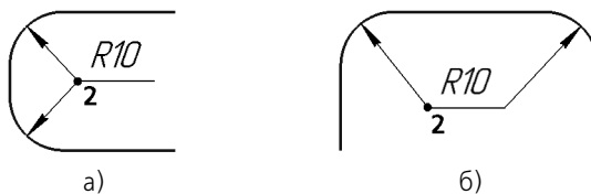
Рис. 129.6. Радиальный размер на полке с ответвлением: а) от начала полки, б) от конца полки.
