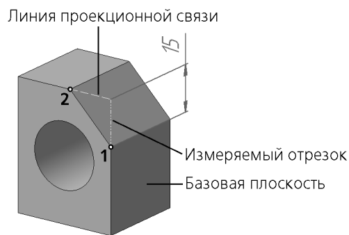
Рис. 64.4. Пример простановки линейного размера
