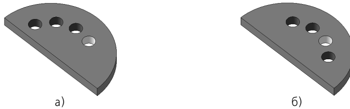
Рис. 52.6. Изменение положения экземпляров в массиве относительно базового экземпляра (базовый экземпляр показан белым цветом): а) базовый экземпляр с номером (1,1); б) базовый экземпляр с номером (1,2)
