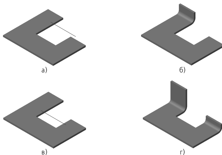
Рис. 38.20. Зависимость результата сгиба от положения линии сгиба: а), в) варианты положения линии сгиба, б), г) соответствующие результаты построения
