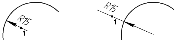
Рис. 129.3. Радиальный размер с автоматически размещенной надписью
