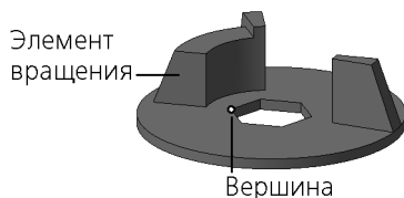
Рис. 24.7. Вращение до вершины
