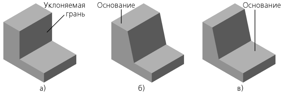
Рис. 30.7. Уклон: а) исходная деталь и уклоняемая грань, б) и в) результат создания уклона в зависимости от выбора основания
