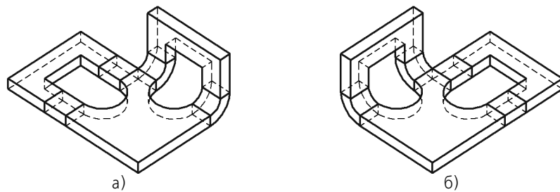
Рис. 40.6. Вырезы, построенные способом По толщине : а) вид детали сразу после создания вырезов, б) результат изменения состояния сгибов
