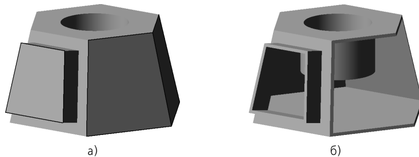
Рис. 30.5. Создание тонкостенной оболочки: а) исходная деталь, удаляемые грани выделены, б) результат создания тонкостенной оболочки
