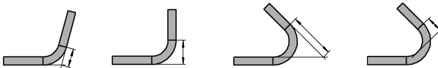
Рис. 38.12. Минимальная длина
