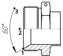
Рис. 130.9. Простановка углового размера с обрывом; способ задания сторон угла — по двум отрезкам
