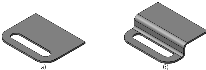
Рис. 38.26. Использование ребра в качестве линии сгиба подсечки: а) расположение ребра, б) результат построения
