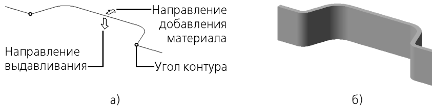
Рис. 36.2. Построение листового тела на основе разомкнутого эскиза: а) эскиз, б) листовое тело
