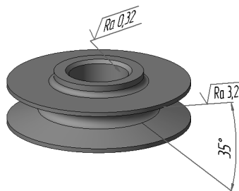
Рис. 65.2. Пример простановки обозначения шероховатости
