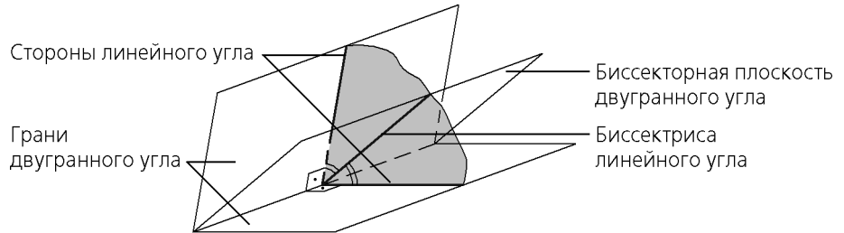
Рис. 59.1. Двугранный угол и его биссекторная плоскость
