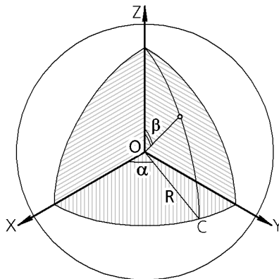
Рис. 45.9. Построение точки по сферическим координатам; XYZ – система координат точки
