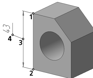
Рис. 64.5. Линейный размер на полке
