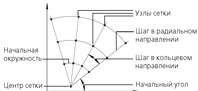
Рис. 138.8. Схема образования концентрической сетки
