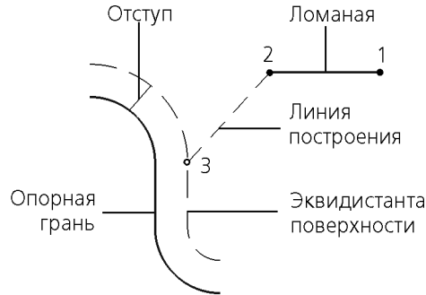
Рис. 46.9. Определение положения вершины путем задания ее смещения от опорной грани
