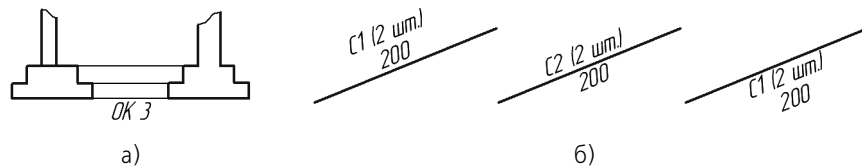
Рис. 134.8. Марка/позиционное обозначение на линии: а) пример использования, б) варианты размещения текста
