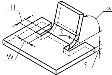
Рис. 35.3. Параметры листового тела
