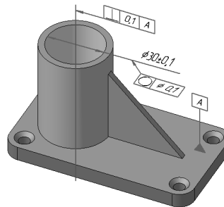
Рис. 65.7. Пример простановки допуска формы и расположения поверхности
