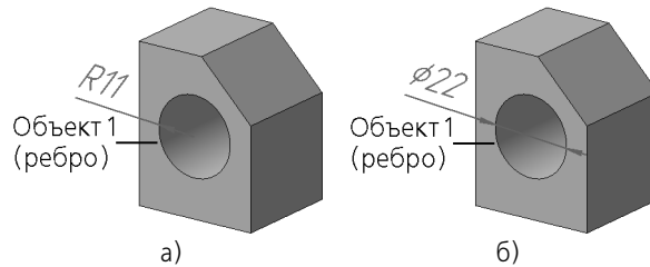
Рис. 64.10. Примеры простановки размеров к ребру детали: а) радиального, б) диаметального
