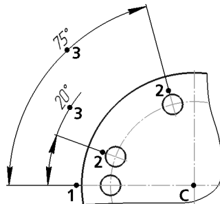
Рис. 130.4. Угловые размеры с ручным размещением размерной надписи; способ задания сторон угла — по двум отрезкам
