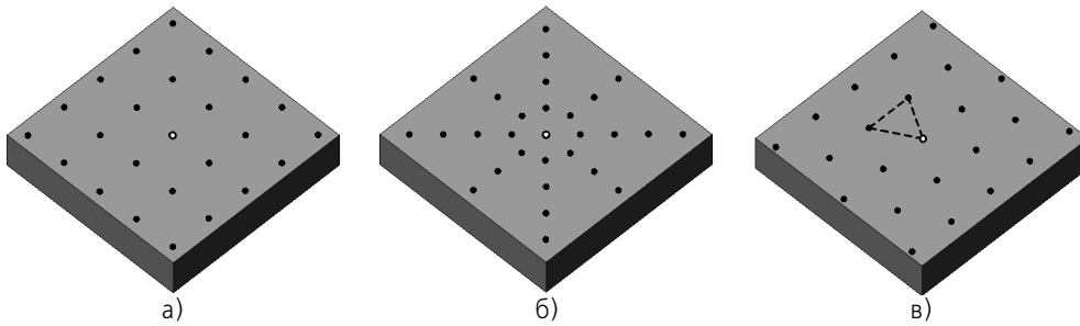
Рис. 45.4. Группа точек, построенная способом По сетке вокруг заданной точки : а) прямоугольная сетка; б) концентрическая сетка; в) гексагональная сетка
