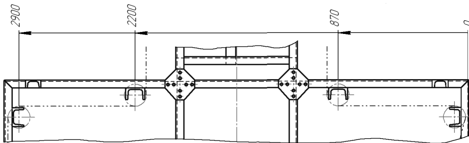
Рис. 128.9. Простановка линейных размеров с общей размерной линией
