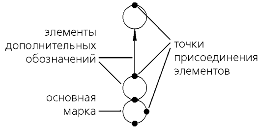
Рис. 134.27. Элементы дополнительных обозначений оси и точки их присоединения
