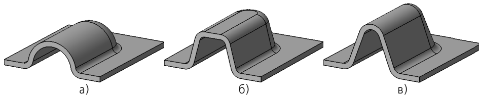
Рис. 42.7. Формы сечения буртиков
