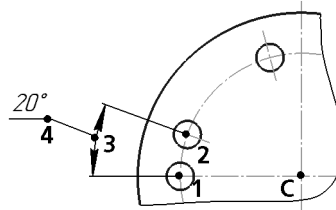
Рис. 130.5. Угловой размер на полке; способ задания сторон угла — по трем точкам
