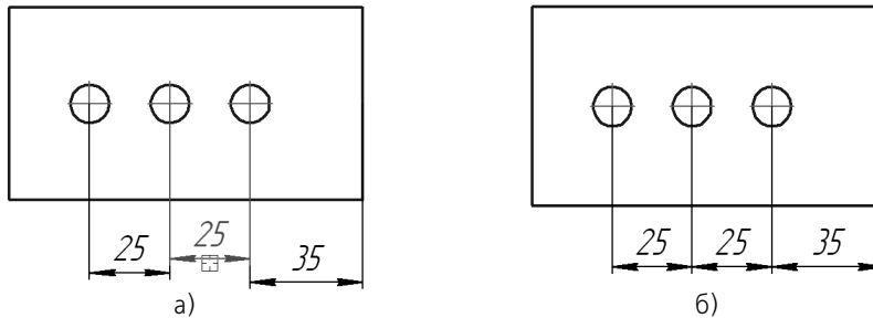
Рис. 127.9. Пример выравнивания линейных размеров: а) указание образца, б) результат выравнивания
