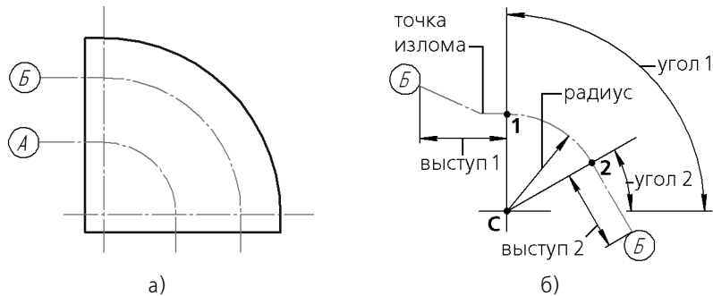
Рис. 134.29. Дуговая координационная ось: а) пример использования, б) параметры оси
