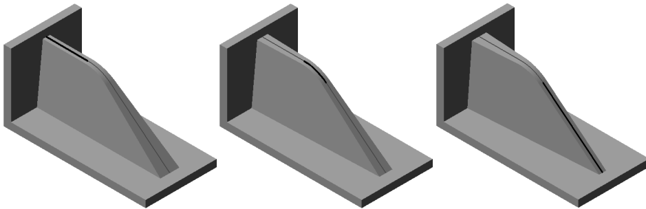
Рис. 30.6. Ребро жесткости с уклоном. Эскиз ребра состоит из трех сегментов. Сегмент, задающий направление уклона, выделен.
