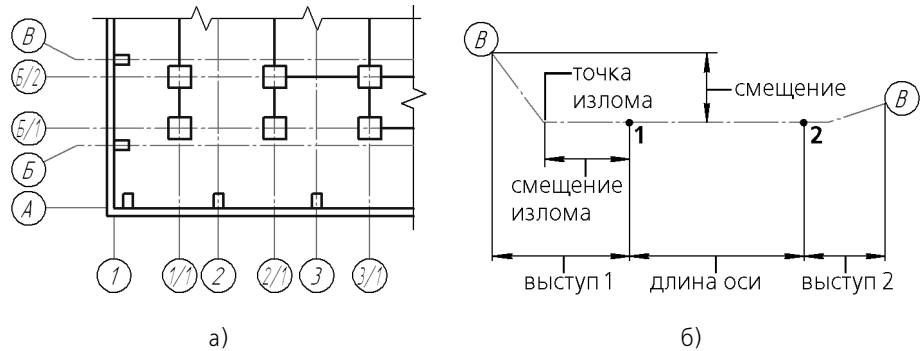
Рис. 134.22. Прямая координационная ось: а) пример использования, б) параметры оси
