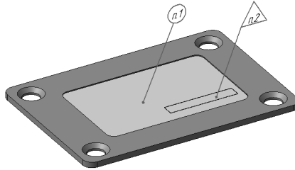
Рис. 65.5. Пример простановки обозначения клеймения
