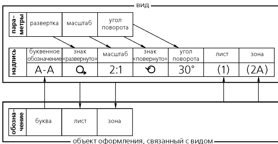
Рис. 149.3. Схема связей между надписью вида и обозначением линии разреза (для машиностроения), связанного с этим видом
