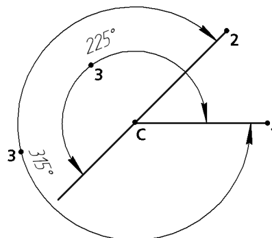
Рис. 130.2. Простановка размера на угол больше 180^\circ между отрезками
