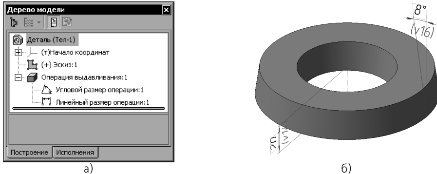
Рис. 64.17. Производные размеры: а) в Дереве построения, б) в окне модели
