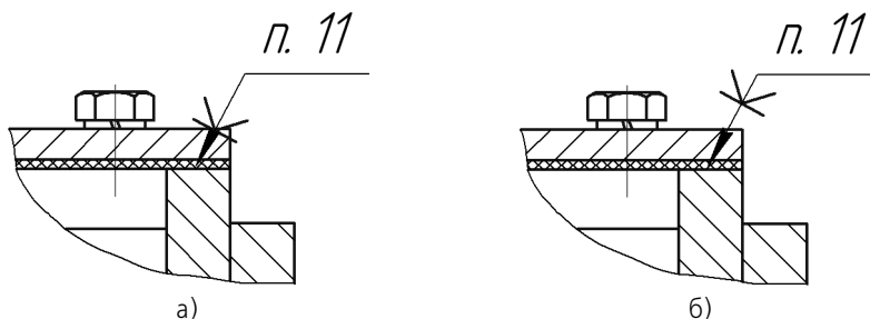
Рис. 133.13. Изменение положения значка на линии-выноске:
