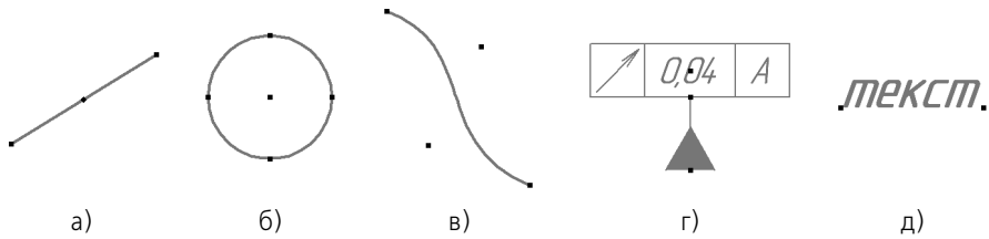
Рис. 136.2. Характерные точки: а) отрезка, б) окружности, в) сплайна, г) допуска формы, д) текста
