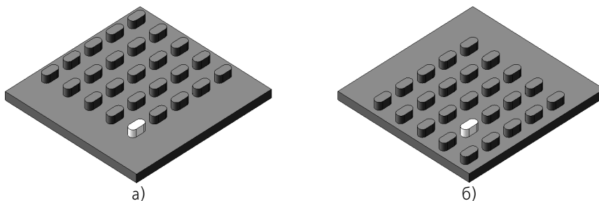
Рис. 51.3. Изменение положения экземпляров в массиве относительно базового (базовый экземпляр показан белым цветом): а) базовый экземпляр с номером (1,1); б) базовый экземпляр с номером (2,2)
