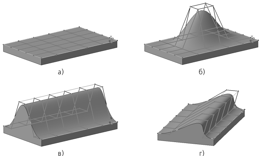
Рис. 49.2. Перемещение полюсов:
