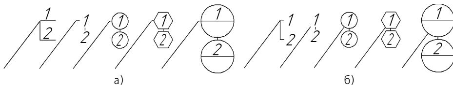
Рис. 133.19. Обозначения позиций различных форм: а) с полкой, б) без полки
