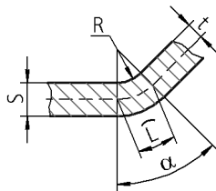
Рис. 35.8. Сечение сгиба плоскостью, перпендикулярной линии сгиба (нейтральная линия показана штрихами)
