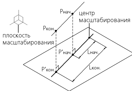
Рис. 49.17. Перемещение полюса при масштабировании в плоскости, плоскостью масштабирования является плоскость XU
