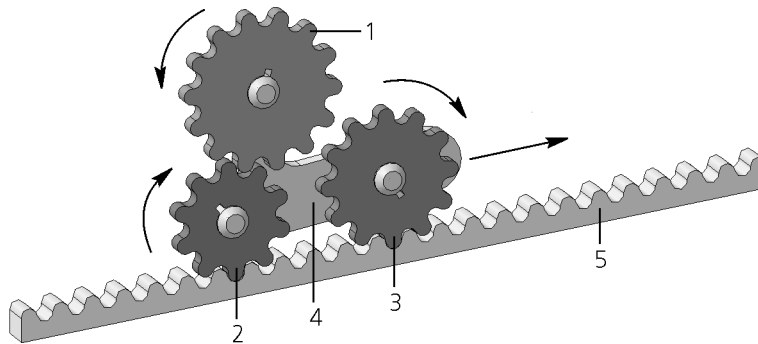
Рис. 79.3. Пример связи перемещений между деталями сборки
