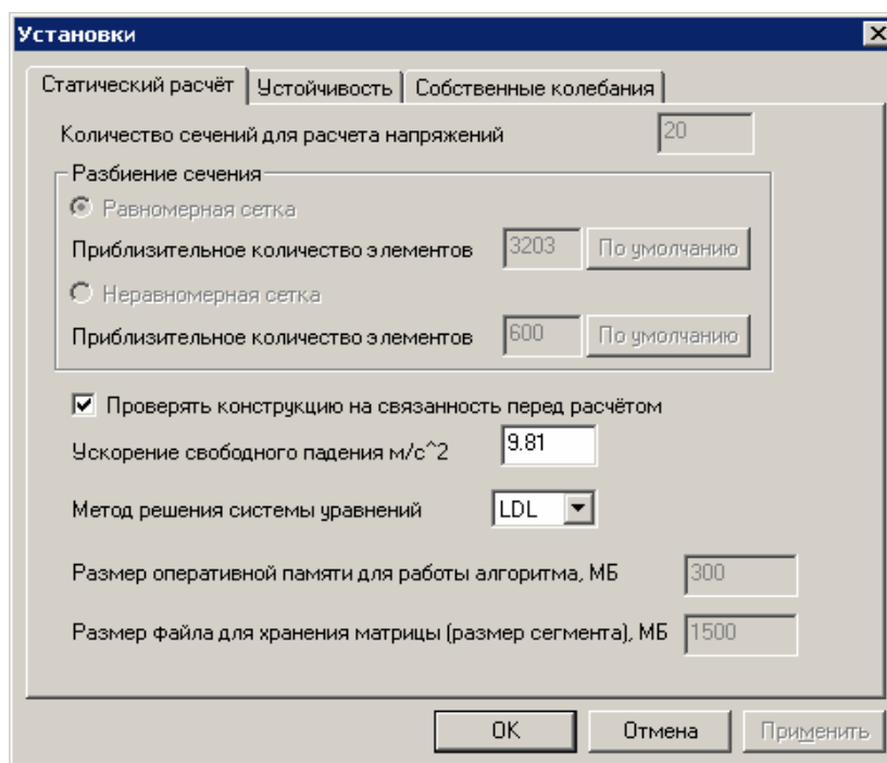
Рис. 2.18 Диалоговое окно Параметры расчета(статический расчёт).
