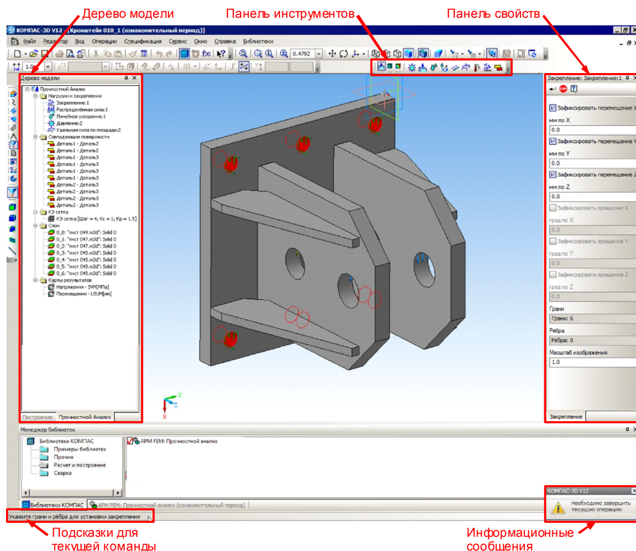
Рис. 1.1 Интерфейс APM FEM.
