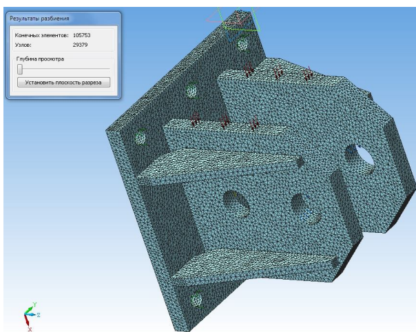
Рис. 2.12 Пример сгенерированной сетки
