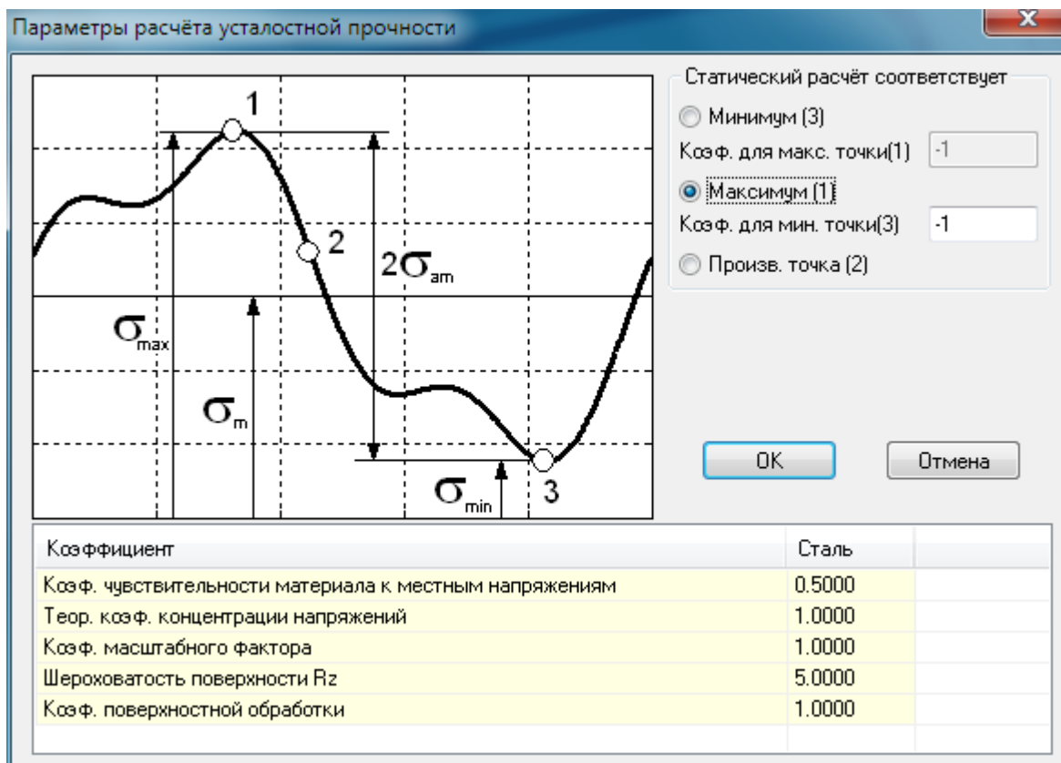
Рис. 2.23 Диалоговое окно Параметры расчёта усталостной прочности.
