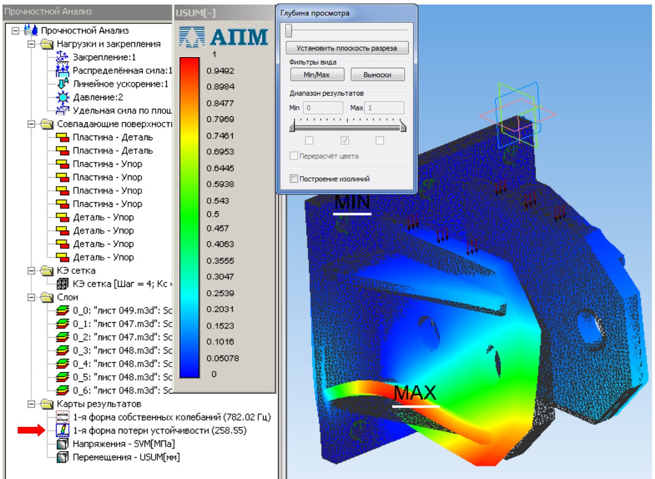
Рис. 2.33 Результаты 1-й формы потери устойчивости
