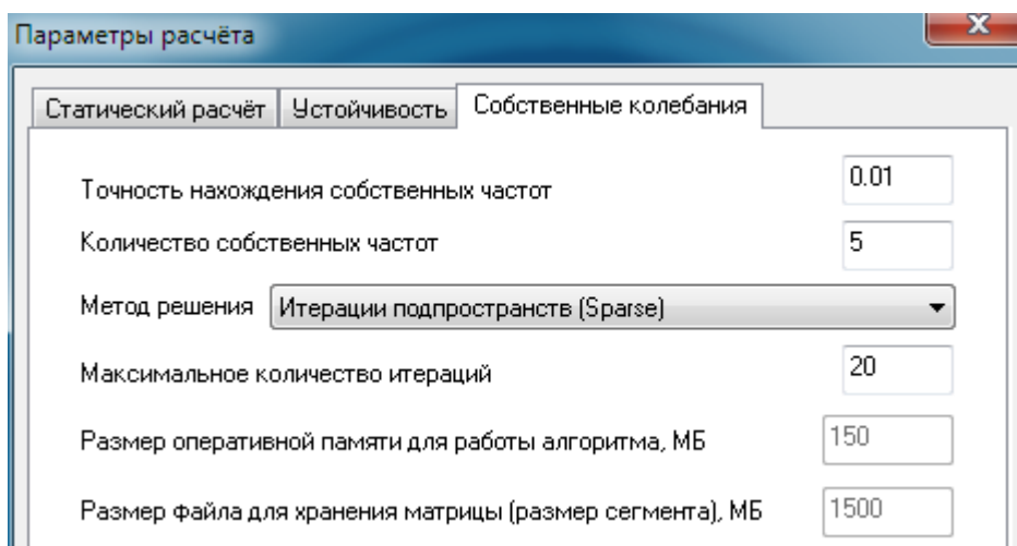
Рис. 2.22 Диалоговое окно Параметры расчета (расчёт собственных колебаний).
