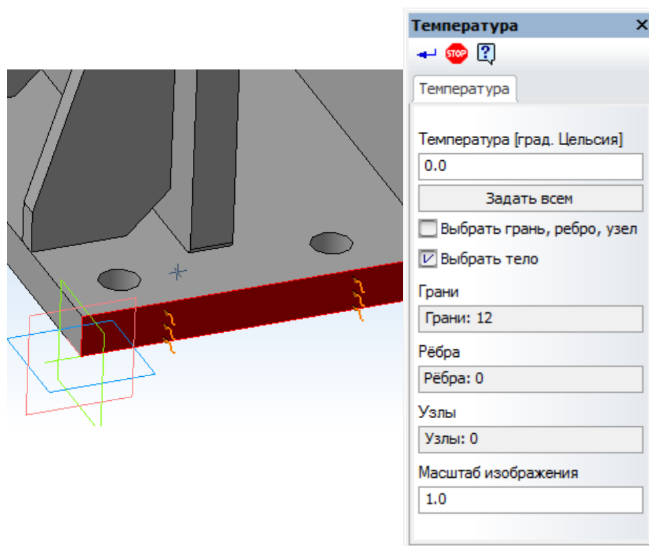
Рис. 2.7 Задание Температуры
