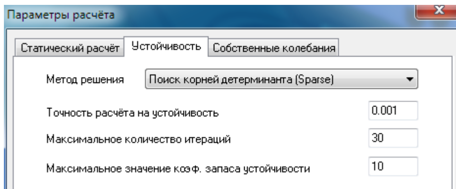
Рис. 2.21 Диалоговое окно Параметры расчета (расчёт устойчивости).
