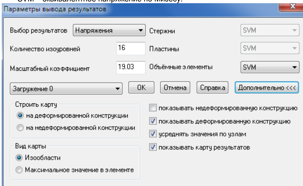
Рис. 2.24 Диалоговое окно Параметры вывода результатов.
