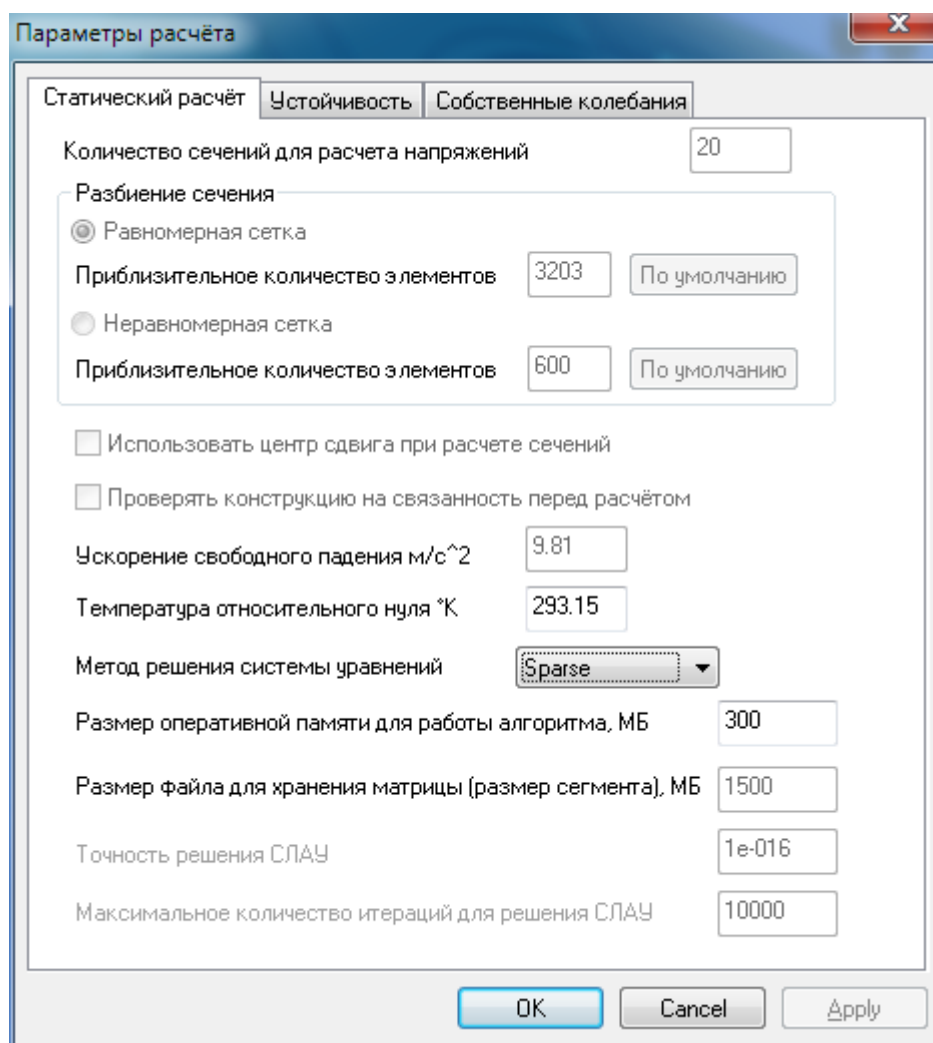
Рис. 2.20 Диалоговое окно Параметры расчета (статический расчёт).
