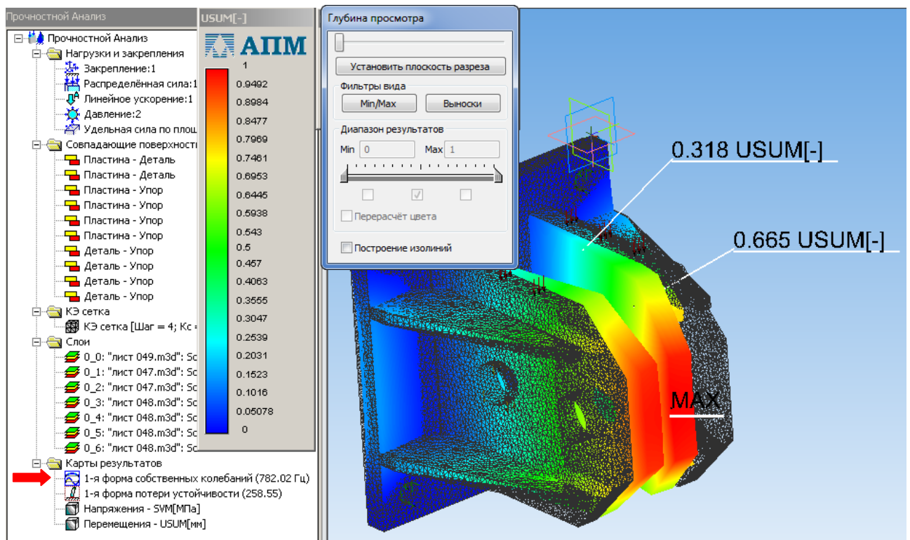
Рис. 2.31 Результаты 1-й формы собственных колебаний.
