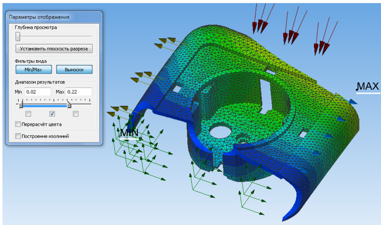
Рис. 2.25 Карта перемещений с заданным диапазоном вывода результатов: показаны только элементы со значениями от 0,02 до 0,22 мм
