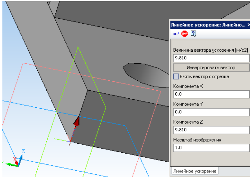
Рис. 2.4 Задание линейного ускорения.
