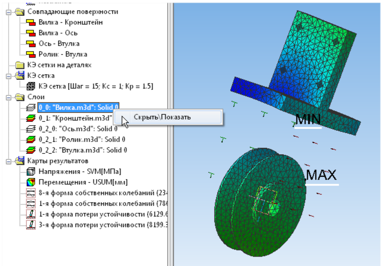
Рис. 2.26 Карта перемещений для сборки с отключёнными слоями
