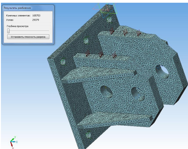
Рис. 2.13 Пример сгенерированной сетки
