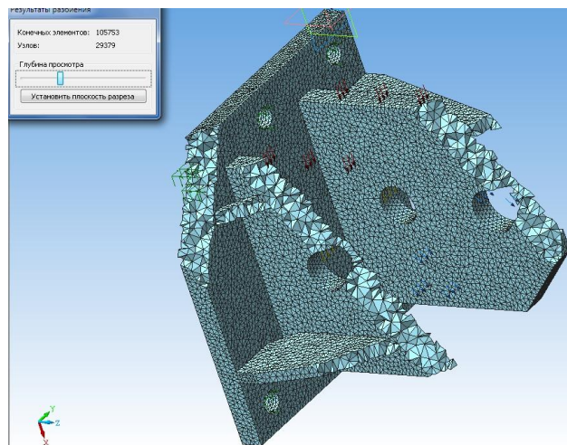
Рис. 2.14 Установка глубины просмотра
