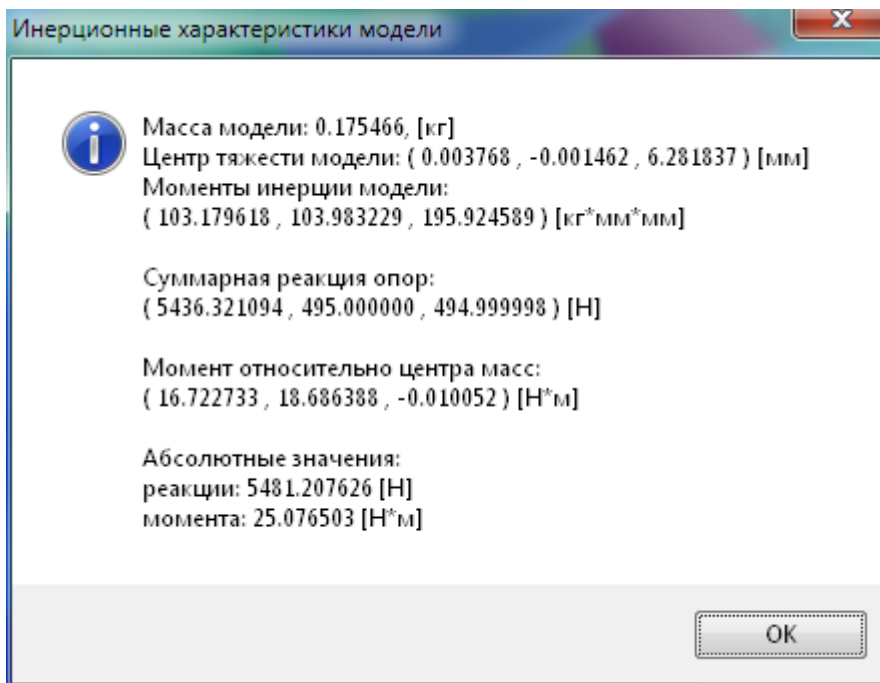
Рис. 2.29 Диалоговое окно Инерционные характеристики модели.
