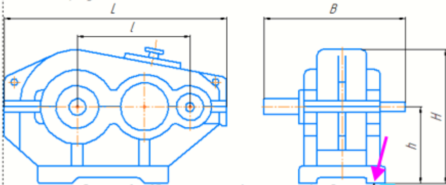
Рисунок 2 – Обозначения основных размеров редуктора
